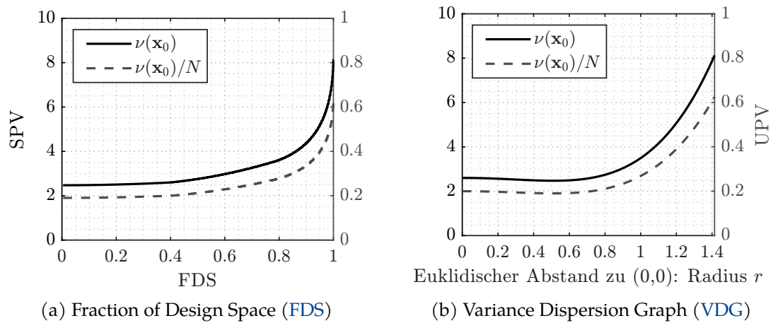
Abbildung 2.9: FDS und VDG für einen CCD mit k = 2 Faktoren.
