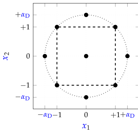
(a) Versuchsplan (CCD)
