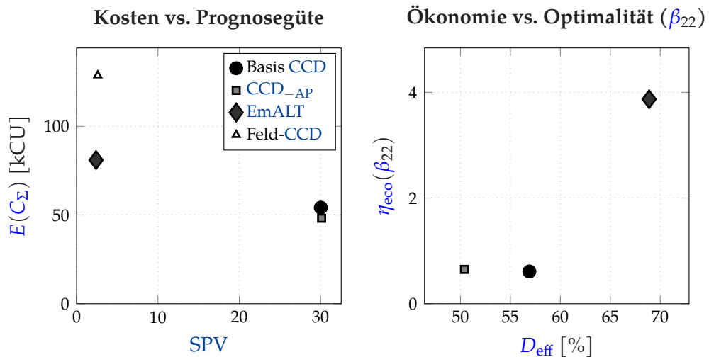
Abbildung 4.23: Links: Exponentieller Zielkonflikt aus Prädiktionsvarianz und Erwartungskosten mit dem EmALT-Design als ökonomischem Optimum. Rechts: Inverse Kausalität zwischen klassischer D-Effizienz und EPI am Beispiel von \beta_{22} (vollständige Evaluation in Anhang B.2).
