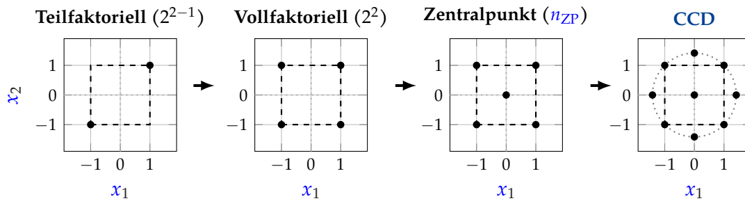
Abbildung 2.8: Strategischer Ansatz zu augmentierter Versuchsplanung für die Lebensdauererprobung nach [50, 51]
