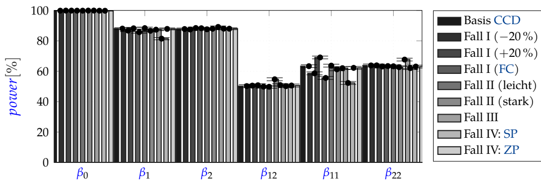
Abbildung B6: Trennschärfe mit 95 %-Konfidenzintervallen in Abhängigkeit der Stör-szenarien für \text{SNR} = 1 .
