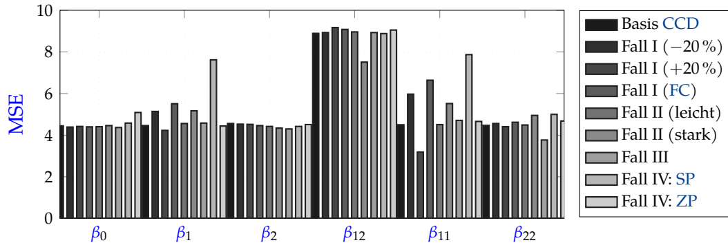
Abbildung B5: Güte der Schätzer (MSE) für \text{SNR} = 1 .
