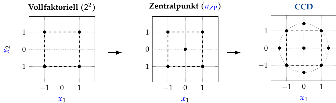
Abbildung 2.3: Strategischer Ansatz zur augmentierten Versuchsplanung für die Lebensdauererprobung nach [42, 43], beispielhaft im zweidimensionalen Fall ( k = 2 ) dargestellt.
