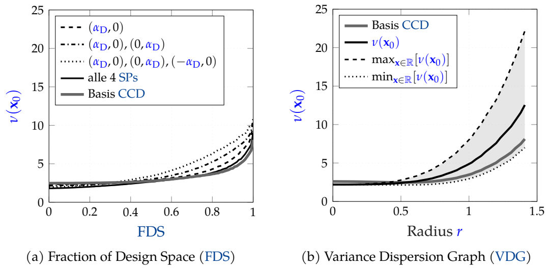
Abbildung 4.8: Vorhersagegüte bei Variation der SP-Anzahl n_{sp} .
