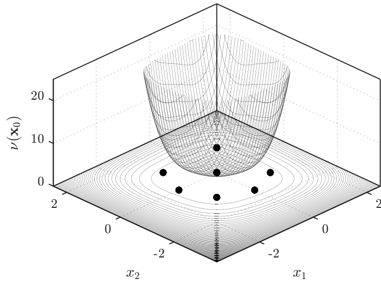
Abbildung 4.9: Dreidimensionale Darstellung der SPV und Konturverlauf für ein asymmetrisches Versuchsdesign.
