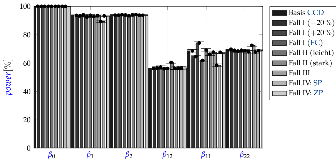
Abbildung 4.5: Trennschärfe mit 95%-Konfidenzintervallen in Abhängigkeit der simulierten Störszenarien.
