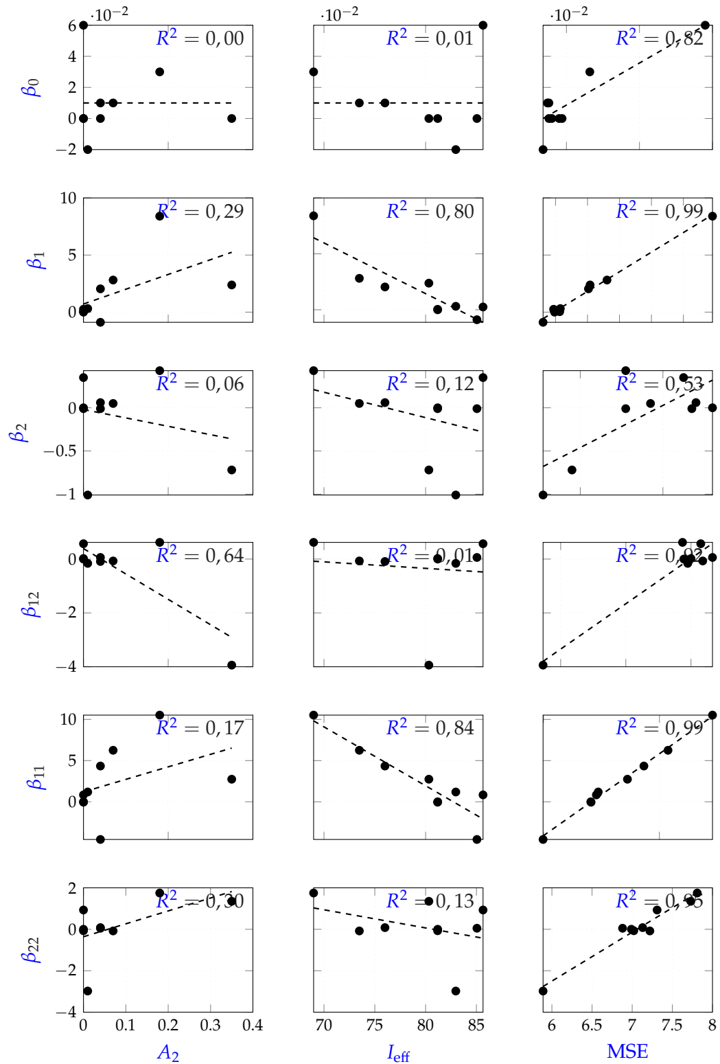
Abbildung B4: Korrelierende Metriken zur prozentualen Trennschärfe-Änderung ( \Delta^{\text{power}} [%]) über alle Koeffizienten und Szenarien ergänzend zu Abbildung 4.6.
