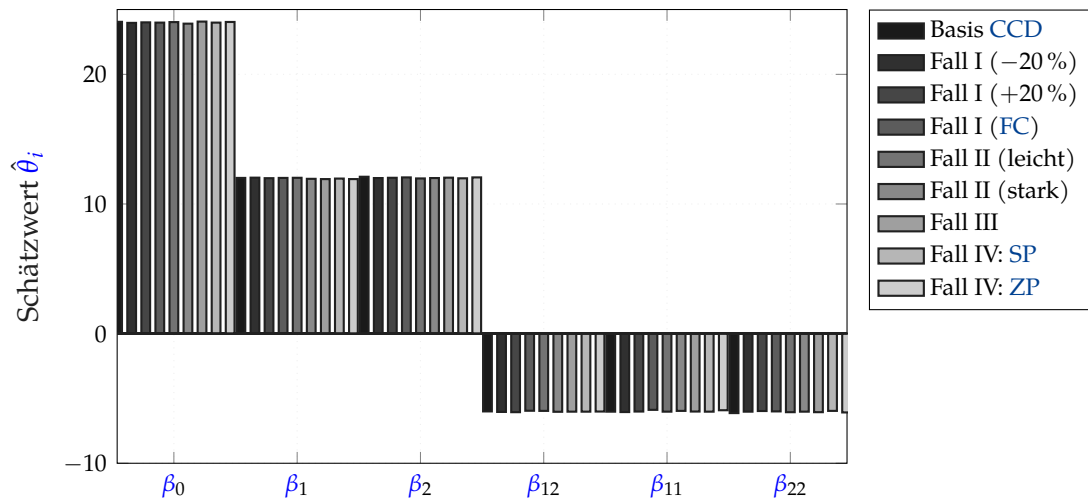
Abbildung 4.4: Absolute Schätzwerte der Modellkoeffizienten für den Arbeitspunkt \text{SNR} = 1,20 . Der Bias bleibt marginal.
