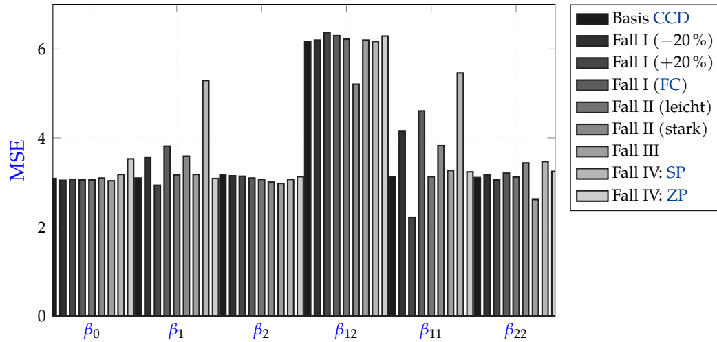
Abbildung 4.3: Güte der Schätzer (MSE) am Arbeitspunkt \text{SNR} = 1,20 . Geometrische Verzerrungen entladen sich primär in der Schätzvarianz (Fall IV: SP).
