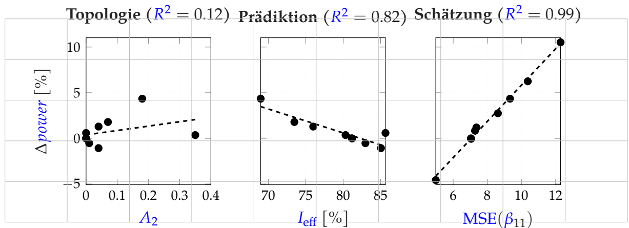
Abbildung 5.7: Korrelation zwischen Design-Metriken und dem resultierenden Trennschärfe-Verlust in den simulierten Störszenarien Fälle I-IV : Durchschnittswerte für alle Koeffizienten in A_2 , I_{eff} , beispielhaft in \beta_{11} und MSE .
