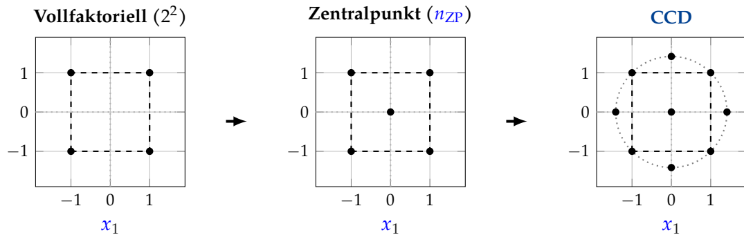
Abbildung 2.3: Strategischer Ansatz zu augmentierter Versuchsplanung für die Lebensdauererprobung nach [42, 43]
