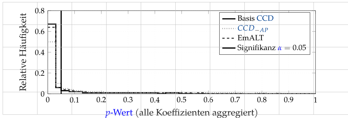
Abbildung 5.16: Relative Häufigkeitsverteilung der p-Werte über alle Simulationssimulationen, welche die numerische Konvergenz und Robustheit der Modellauswertung bestätigt.
