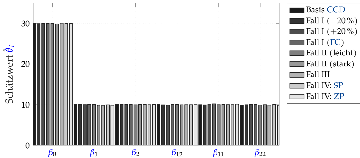
Abbildung 5.2: Absolute Schätzwerte der Modellkoeffizienten für den Arbeitspunkt \text{SNR} = 1,33 .
