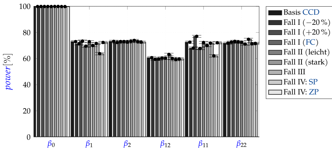
Abbildung 5.4: Trennschärfe mit 95 %-Konfidenzintervallen in Abhängigkeit der Störszenarien. Trotz kritischer Parameterkonstellation ( \text{SNR} = 1,33 ) bleiben die power -Verluste bei Erhalt der Symmetrie gering.
