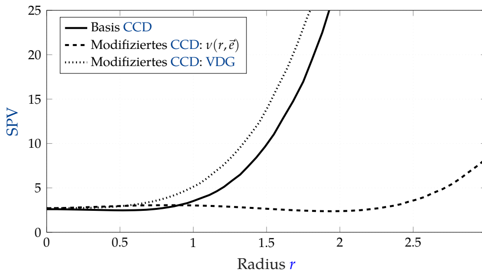
Abbildung 5.14: Der klassische VDG verschleiert den lokalen Design-Nutzen des um APs modifizierten CCD durch radiale Mittelung. Der EVG belegt hingegen die signifikante SPV -Reduktion zielgerichtet entlang des Extrapolationsvektors zum Prognosepunkt.
