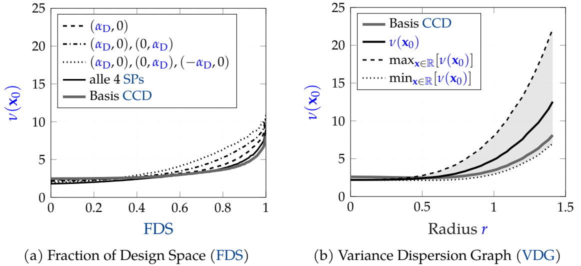
Abbildung 5.10: Vorhersagegüte bei Variation der SP-Anzahl n_{SP} für einen CCD mit k = 2 Faktoren. SPV-Werte für verschiedene Varianten entfallener Sternpunkte. Abbildung 5.10b zeigt den Fall des vollständigen Entfalls der Sternpunkte (\alpha_D; 0) und (0; \alpha_D) im Hochlastbereich.
