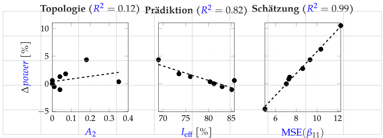
Abbildung 5.7: Korrelation zwischen Design-Metriken und dem resultierenden Trennschärfe-Verlust in den simulierten Störszenarien Fälle I-IV : Durchschnittswerte für alle Koeffizienten in A_2 , I_{\text{eff}} , beispielhaft in \beta_{11} und MSE .
