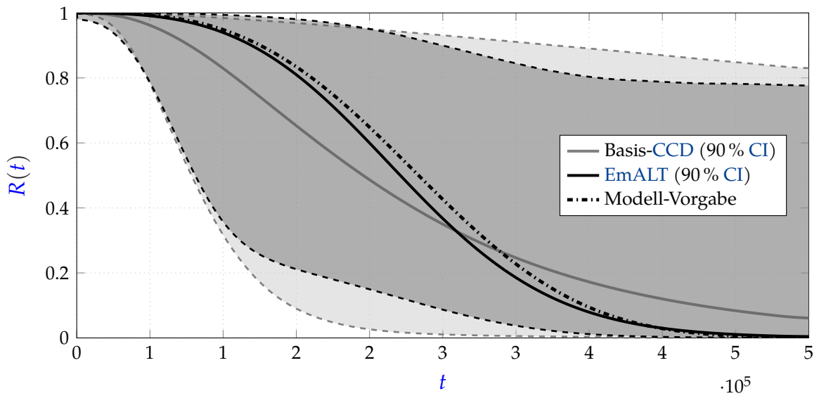
Abbildung 5.24: Vergleich der prognostizierten Überlebenswahrscheinlichkeit R(t) am Feldbetriebspunkt inklusive 90 %-CI. Aufgrund der Distanz weisen beide Designs hohe Prognoseunsicherheiten auf, das EmALT-Design (schwarz) reproduziert das wahre Zuverlässigkeitsmodell jedoch mit stellenweise geringerer Varianz als das Basis-CCD (grau).
