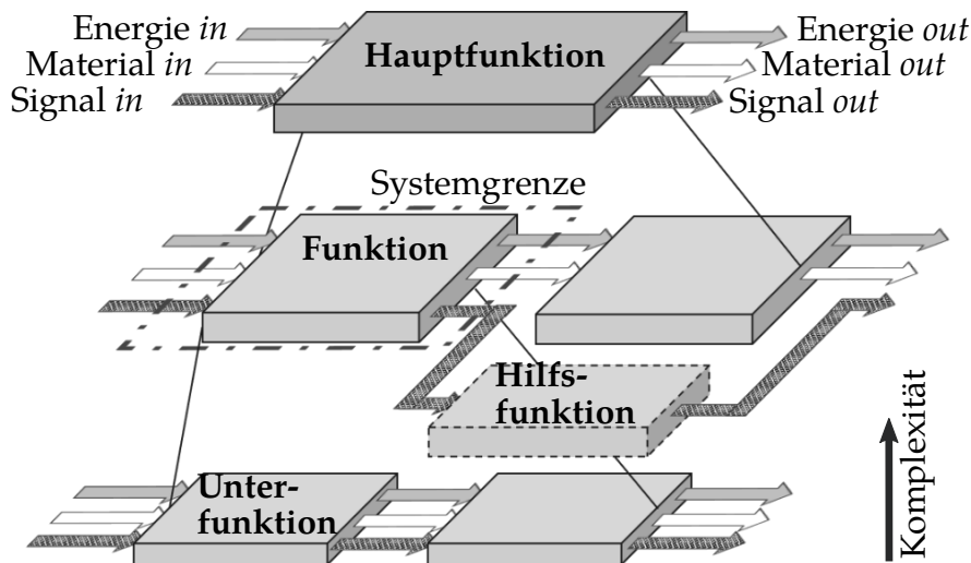
Abbildung 4.1: FBD mit Haupt-, Neben- und Teilfunktionen zur lückenlosen Identifikation funktionskritischer Einflussgrößen (in Anlehnung an [97] nach [99]).
