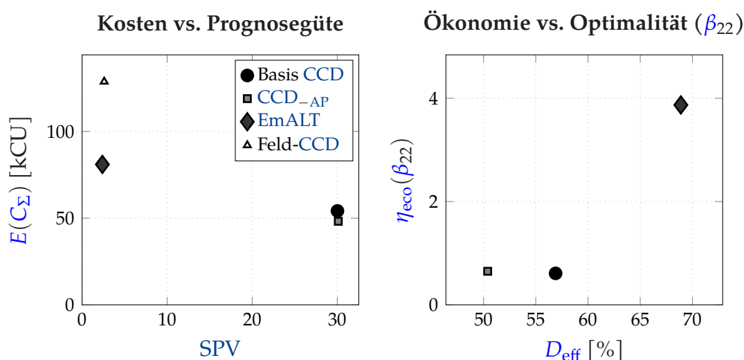
Abbildung 5.23: Links: Exponentieller Zielkonflikt aus Prädiktionsvarianz und Erwartungskosten mit dem EmALT -Design als ökonomischem Optimum. Rechts: Inverse Kausalität zwischen klassischer D -Effizienz und EPI am Beispiel von \beta_{22} (vollständige Evaluation in Anhang B.2).
