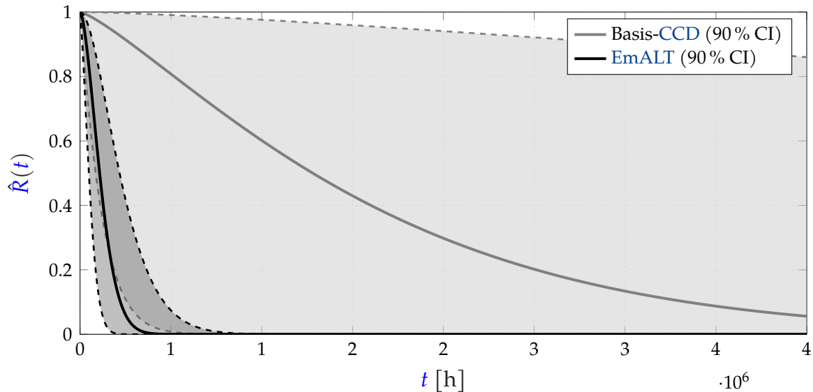
Abbildung 6.4: Empirische Lebensdauerprognose am Feldpunkt. Das EmALT -Design liefert eine radikal verkleinerte Prädiktionsvarianz (schmales Konfidenzband). Sein Median verbleibt kohärent innerhalb des weiten Vertrauensbereichs des Basis- CCD , zeichnet jedoch ein realitätsnäheres und konservativeres Ausfallverhalten.
