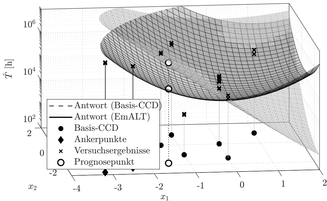
Abbildung 6.2: Modellanpassung im Parameterraum (logarithmische Darstellung): Beide Regressionsflächen im direkten visuellen Vergleich. Das Basis- CCD extrapoliert starr aus dem Hochlastzentrum. Das EmALT -Design wird durch die APs im südwestlichen Parameterbereich gestützt und erfährt eine merkliche Dämpfung der prognostizierten Lebensdauer.
