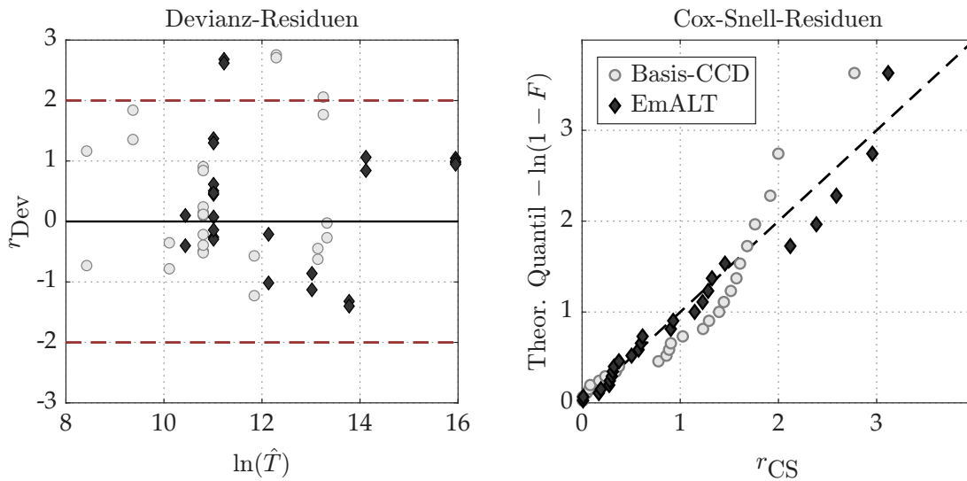
Abbildung 6.3: Residuenanalyse der Modellpassung für das Basis-CCD und das EmALT-Design am realen Prüfstandsdatensatz ( N = 26 ): Standardisierte Devianz-Residuen über \ln(\hat{T}) (links) sowie Cox-Snell-Residuen (rechts).
