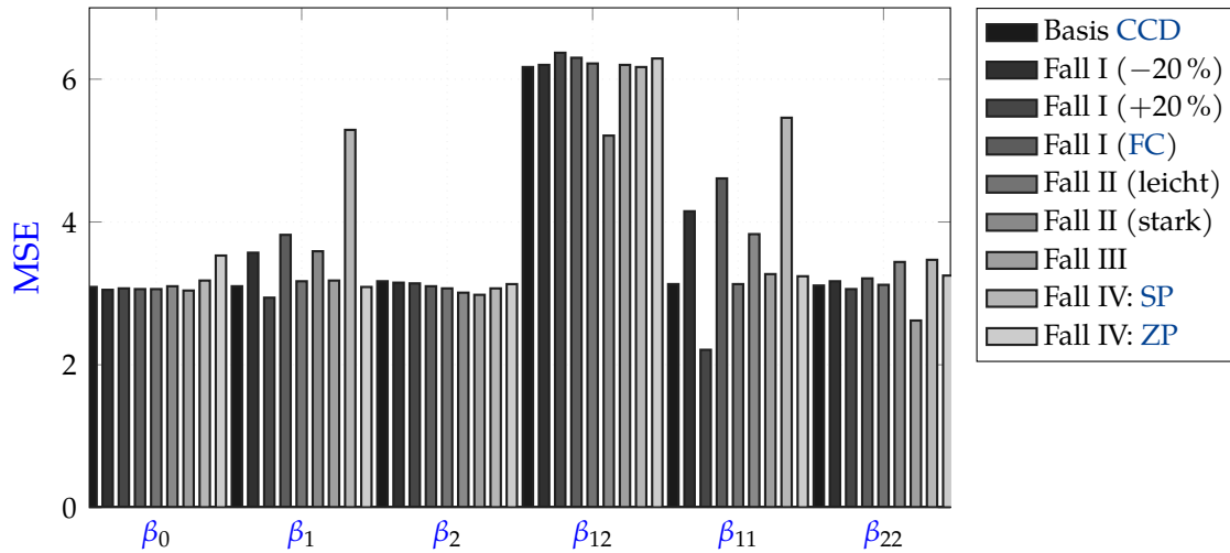
Abbildung 5.2: Güte der Schätzer ( MSE ) am Arbeitspunkt SNR = 1,20 . Geometrische Verzerrungen entladen sich primär in der Schätzvarianz, insbesondere beim Wegfall von Rand-Freiheitsgraden durch asymmetrische Ausfälle ( Fall IV: SP ).
