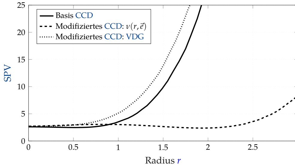
Abbildung 5.14: Der klassische VDG verschleiert den lokalen Design-Nutzen des um APs modifizierten CCD durch radiale Mittelung. Der EVG belegt hingegen die signifikante SPV -Reduktion zielgerichtet entlang des Extrapolationsvektors zum Prognosepunkt.
