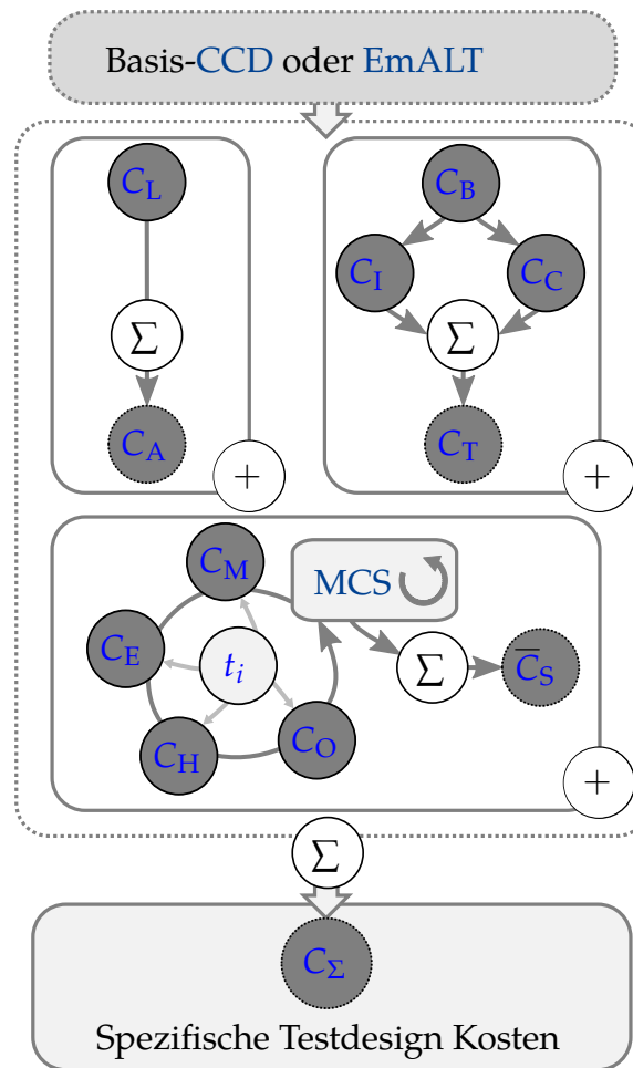
Abbildung 5.15: Struktur des Kostenmodells zur Berechnung der Gesamtkosten C_\Sigma als Funktion der Versuchsplan-Implementierung, identifizierter Kostenfaktoren sowie zufallsbehafteter Versuchslaufzeiten t_i (in Anlehnung an [95]).
