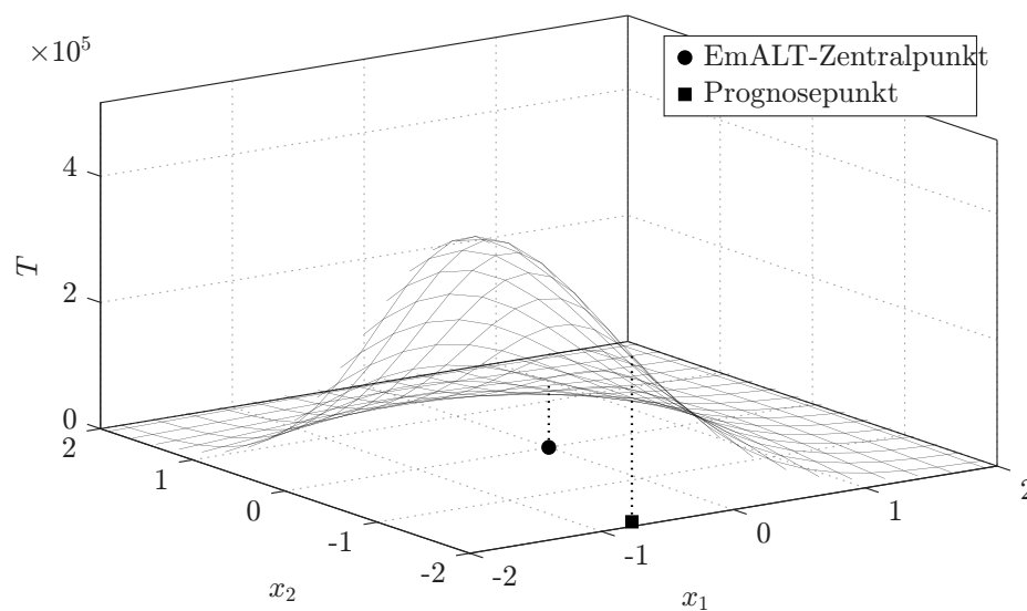
Abbildung 5.16: Antwortfläche der charakteristischen Systemlebensdauer T in Abhängigkeit der Faktoren x_1 und x_2 . Die Projektion verdeutlicht die massive Extrapolationsdistanz zwischen dem DoE-Zentrum und den geforderten Feld-Bedingungen.
