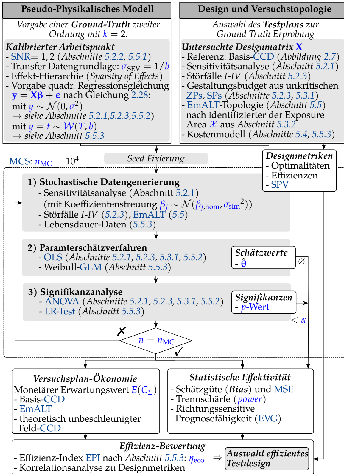
Abbildung 5.1: Methodische Architektur der Monte-Carlo-Simulationsumgebung zur ganzheitlichen stochastisch-ökonomischen Bewertung multivariater Lebensdauertests für sämtliche Abschnitte in Kapitel 5.
