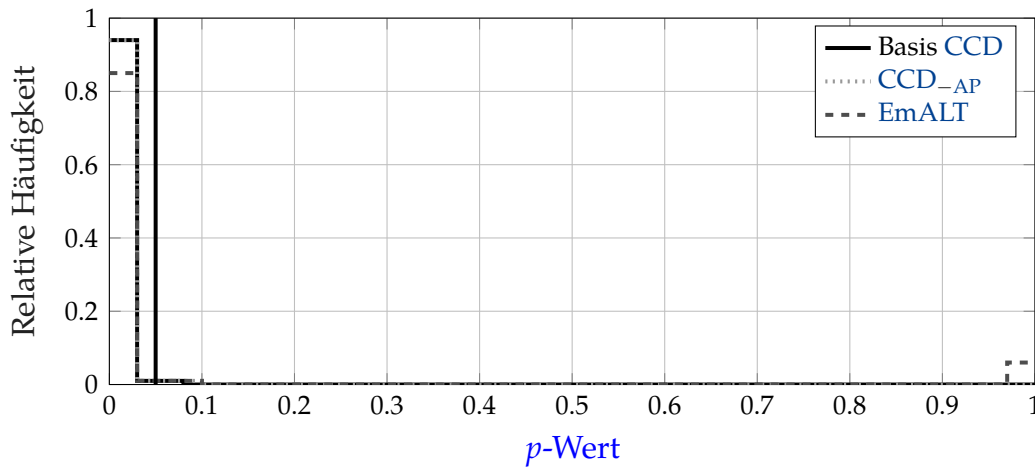
Abbildung 5.21: Aggregierte p -Wert Histogramme der MLE-Signifikanztests. Die stochastische Auswertung liefert artefaktfreie Verteilungen.
