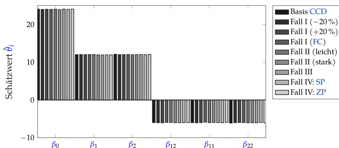
Abbildung 5.3: Absolute Schätzwerte der Modellkoeffizienten für den Arbeitspunkt \text{SNR} = 1,20 . Der Bias bleibt marginal; die OLS-Schätzung ist fundamental erwartungstreu.
