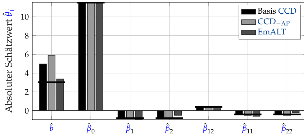
Abbildung 5.20: Absolute Schätzwerte der MLE-Koeffizienten im Weibull-Modell ( \text{SNR} = 1,20 ). Der Schätzwert der Basislebensdauer \hat{\beta}_0 bleibt exakt; die Terme höherer Ordnung spiegeln die durch die Multikollinearität induzierte Varianzumverteilung wider.
