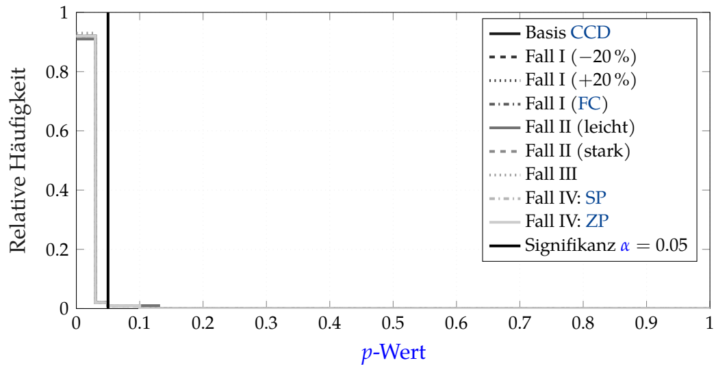
Abbildung 5.7: p -Wert Histogramm für den Signifikanztest am Beispiel von \beta_2 . Die kumulierte Häufigkeit links der \alpha = 0,05 -Schranke entspricht der berechneten power .
