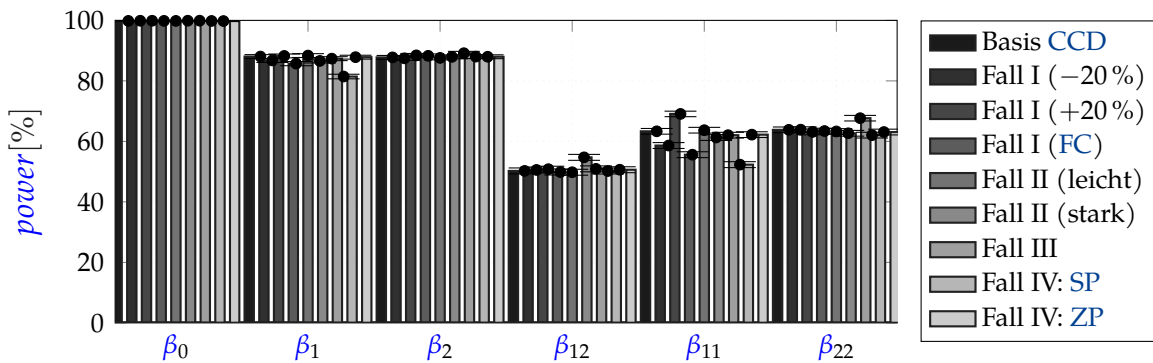
Abbildung B6: Trennschärfe mit 95 %-Konfidenzintervallen in Abhängigkeit der Störszenarien für \text{SNR} = 1 .
