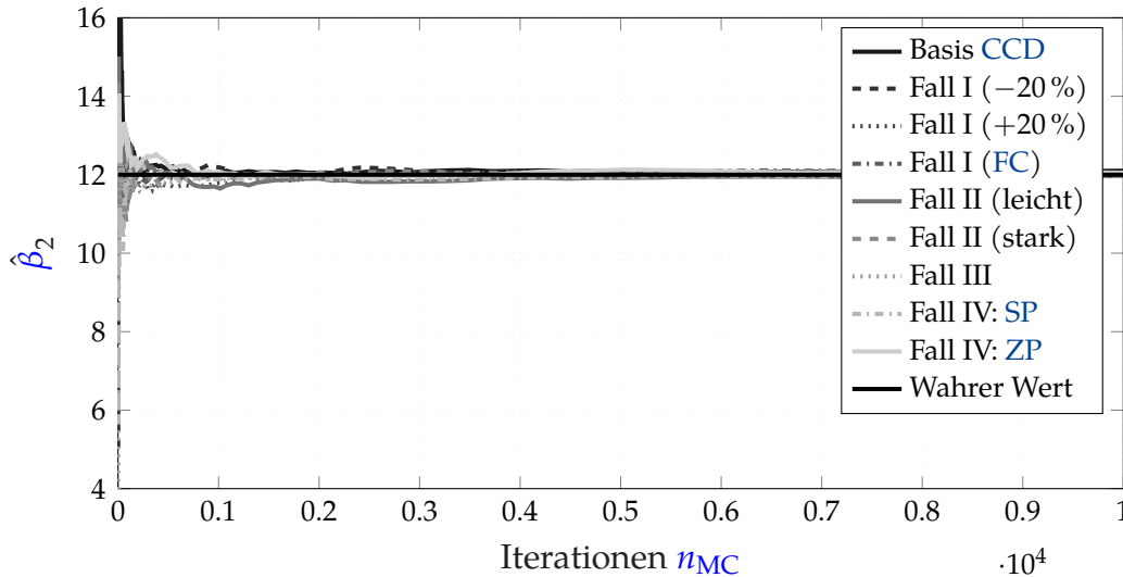
Abbildung 5.4: Numerische Konvergenz am Beispiel des Schätzwertes zu \hat{\beta}_2 über die MCS-Iterationen.
