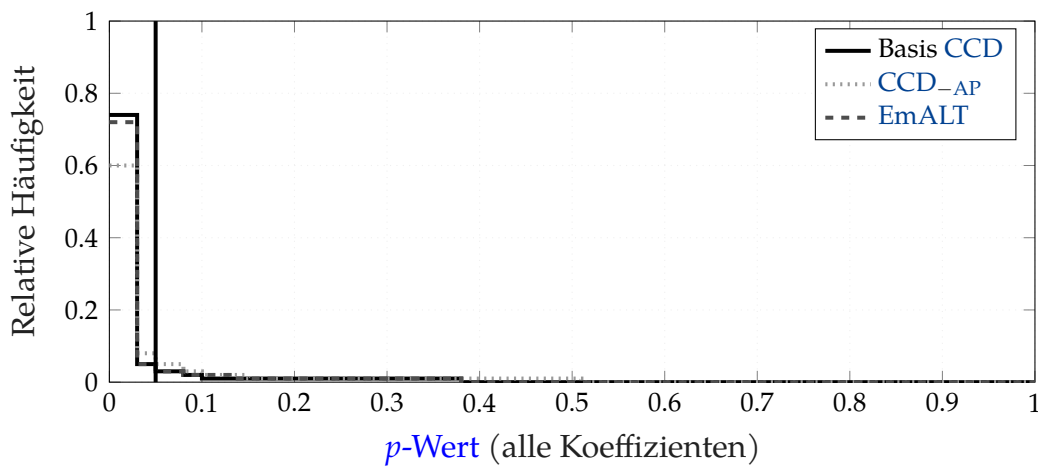
Abbildung 5.18: Aggregierte p -Wert Histogramme der verglichenen Designvarianten. Der konforme Verlauf belegt die Abwesenheit systematischer Verzerrungen in der Signifikanzprüfung.
