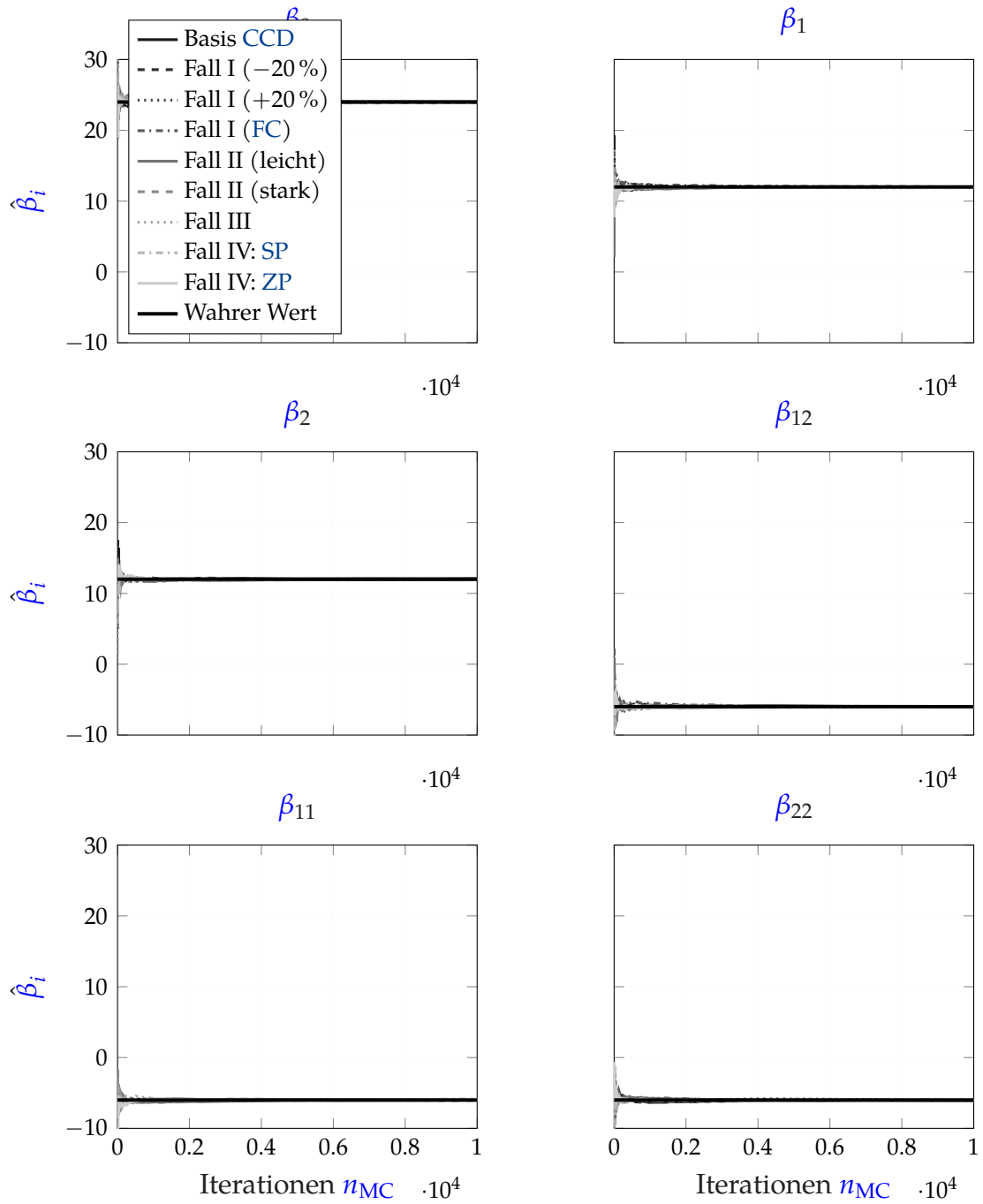
Abbildung B2: Konvergenz der OLS-Parameterschätzwerte ( \hat{\beta}_i ). Alle Modelle erweisen sich unabhängig von der geometrischen Verzerrung als erwartungstreu. Die Schätzungen stabilisieren sich bei der n_{MC} = 10^4 reproduzierbar.
