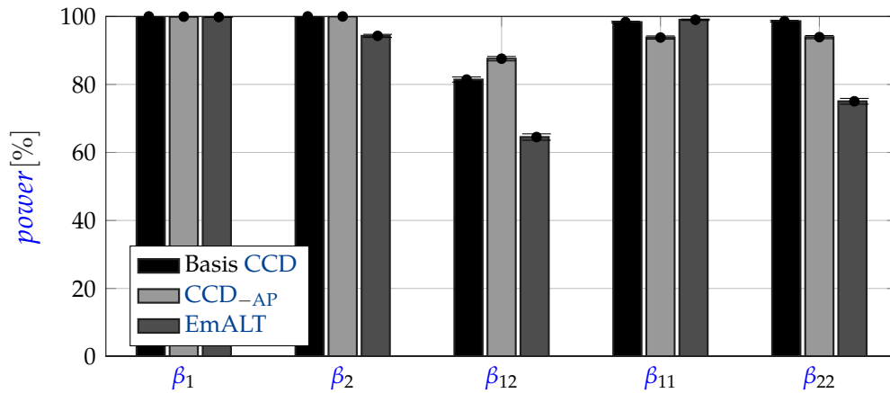
Abbildung 5.22: Vergleichende Analyse der MLE-power. Das EmALT-Design rettet die für die Modellierung essenziellen Terme vor dem vollständigen Zusammenbruch.
