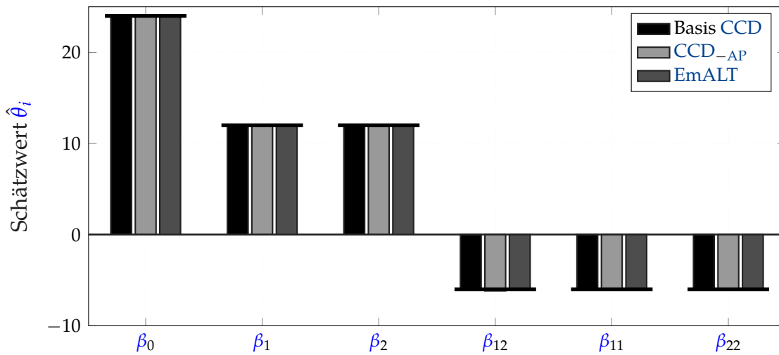
Abbildung 5.17: Absolute Schätzwerte der Modellkoeffizienten für die asymmetrischen Designvarianten am Arbeitspunkt \text{SNR} = 1,20 . Der Bias bleibt marginal; die Erwartungstreue des OLS-Schätzers ist gewahrt.
