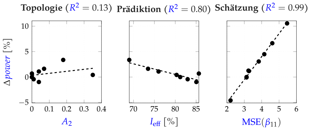
Abbildung 5.8: Korrelation zwischen a priori Design-Metriken und dem resultierenden Trennschärfe-Verlust in den Störszenarien: Der MSE übersetzt den geometrischen Fehler am direktesten in die probabilistische Trennschärfe.
