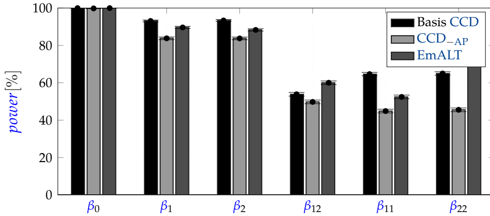
Abbildung 5.19: Vergleichende Analyse der absoluten statistischen Trennschärfe. Die asymmetrische Extrapolationsabsicherung (EmALT) stellt die Detektionsrate im Vergleich zur reinen Ausdünnung nahezu vollständig wieder her.
