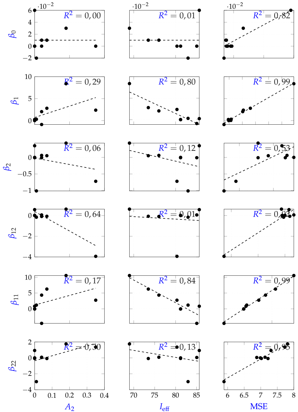
Abbildung C5: Korrelierende Metriken zur prozentualen Trennschärfe-Änderung ( \Delta power [%]) über alle Koeffizienten und Szenarien ergänzend zu Abbildung 5.7.
