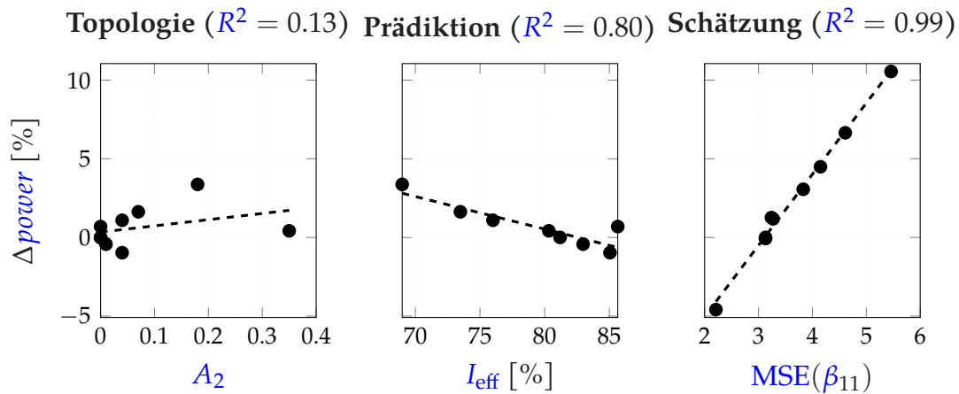
Abbildung 5.7: Korrelation zwischen Design-Metriken und dem resultierenden Trennschärfe-Verlust in den simulierten Störszenarien Fälle I-IV : Durchschnittswerte für alle Koeffizienten in A_2 , I_{\text{eff}} , beispielhaft in \beta_{11} und MSE .
