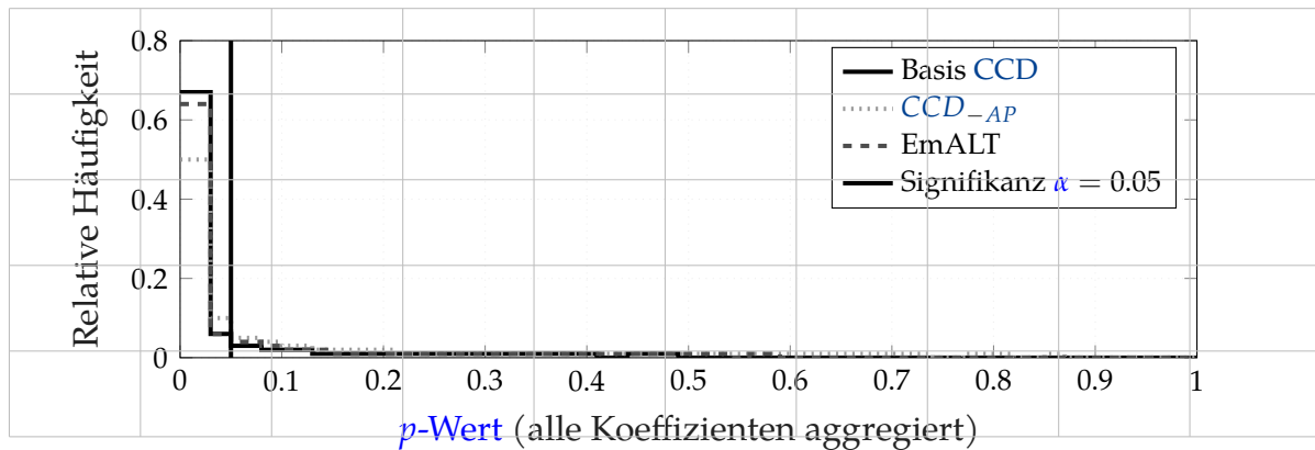
Abbildung 5.16: Relative Häufigkeitsverteilung der p-Werte über alle Simulationsiterationen, welche die numerische Konvergenz und Robustheit der Modellauswertung bestätigt.
