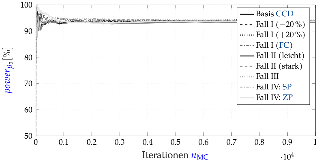
Abbildung 5.5: Numerische Konvergenz der Trennschärfe über die Simulationsläufe am Beispiel von \beta_2 .
