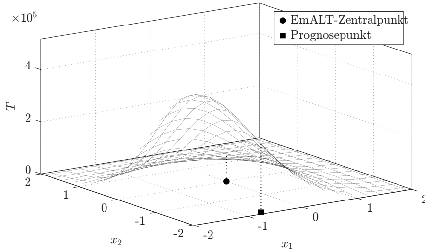
Abbildung 4.16: Antwortfläche der charakteristischen Systemlebensdauer T .
