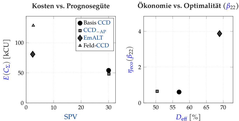
Abbildung 4.20: Exponentieller Zielkonflikt aus Prädiktionsvarianz und Erwartungskosten sowie die inverse Kausalität zwischen D -Effizienz und EPI .
