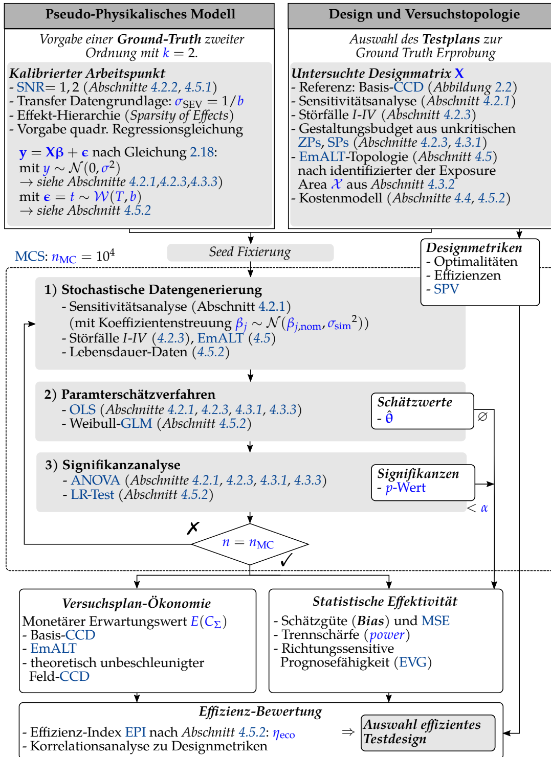
Abbildung 4.1: Methodische Architektur der Monte-Carlo-Simulationsumgebung. Das Framework fungiert als struktureller Fahrplan für die Validierung der statistischen Effektivität und ökonomischen Effizienz.
