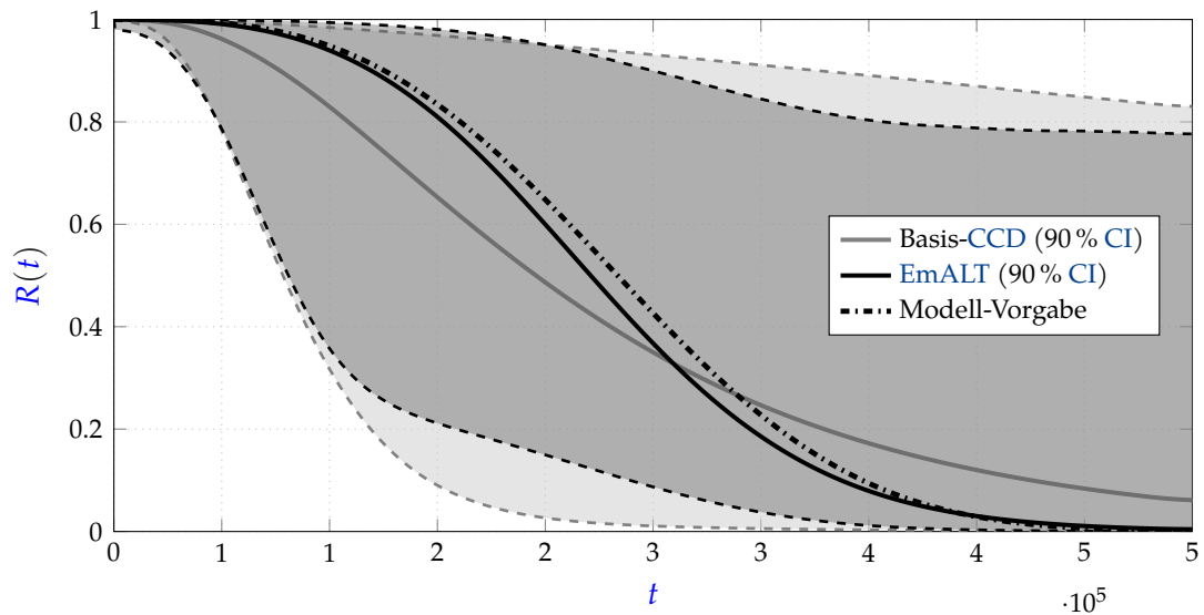
Abbildung 4.21: Vergleich der prognostizierten Überlebenswahrscheinlichkeit R(t) am Feldbetriebspunkt inklusive 90 %-CI.
