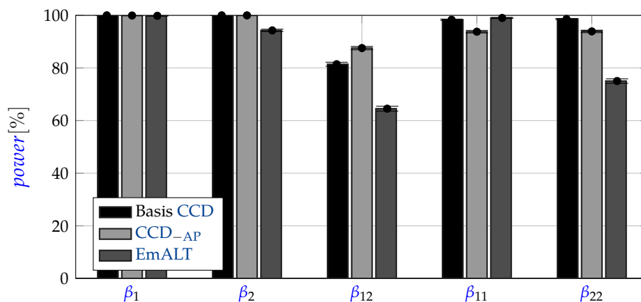
Abbildung 4.19: Vergleichende Analyse der MLE-power.
