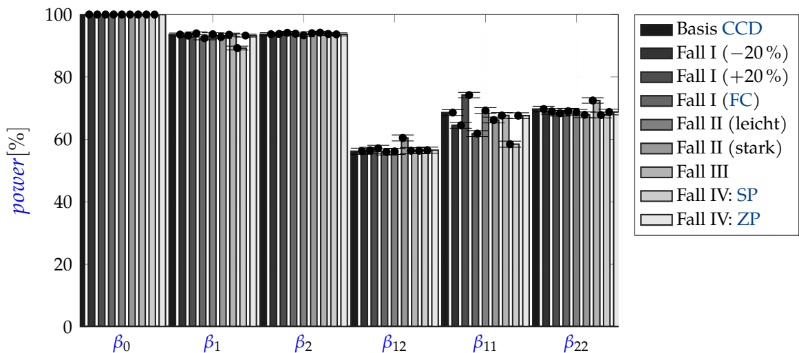
Abbildung 5.4: Trennschärfe mit 95 %-Konfidenzintervallen in Abhängigkeit der simulierten Störszenarien ( SNR = 1,20 ). Bei Erhalt der Basissymmetrie bleiben die power -Verluste bemerkenswert gering.
