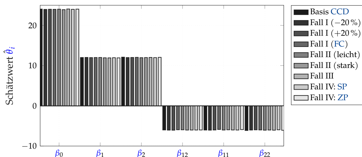
Abbildung 5.2: Absolute Schätzwerte der Modellkoeffizienten für den Arbeitspunkt \text{SNR} = 1,20 . Der Bias bleibt marginal; die OLS-Schätzung ist erwartungstreu.
