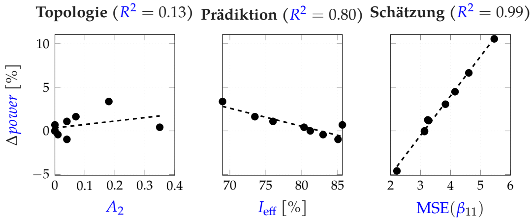
Abbildung 5.7: Korrelation zwischen Design-Metriken und dem resultierenden Trennschärfe-Verlust in den Störszenarien: Der MSE übersetzt den geometrischen Fehler am direktesten in die probabilistische Trennschärfe.
