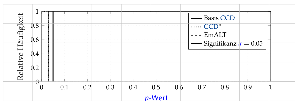
Abbildung 5.19: Relative Häufigkeitsverteilung der p-Werte (Weibull-Modell), welche die numerische Konvergenz und Robustheit der MLE -Auswertung bestätigt.
