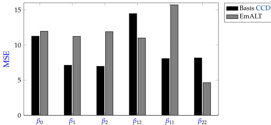
Abbildung 5.18: Güte der Schätzer ( MSE ). Der durch den Wegfall der Sternpunkte induzierte Varianzanstieg wird durch die strategische Positionierung der Ankerpunkte im EmALT effektiv abgefedert.
