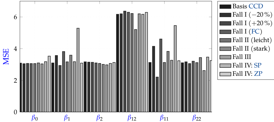
Abbildung 5.1: Güte der Schätzer (MSE) am Arbeitspunkt \text{SNR} = 1,20 . Geometrische Verzerrungen entladen sich primär in der Schätzvarianz, insbesondere beim Wegfall von Rand-Freiheitsgraden durch asymmetrische Ausfälle ( Fall IV: SP ).
