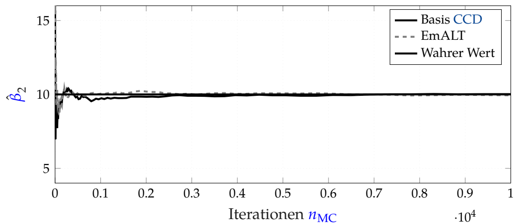
Abbildung 5.16: Numerische Konvergenz der Schätzwerte über die Monte-Carlo-Iterationen, stellvertretend für die methodische Stabilität der asymmetrischen Auswertung.
