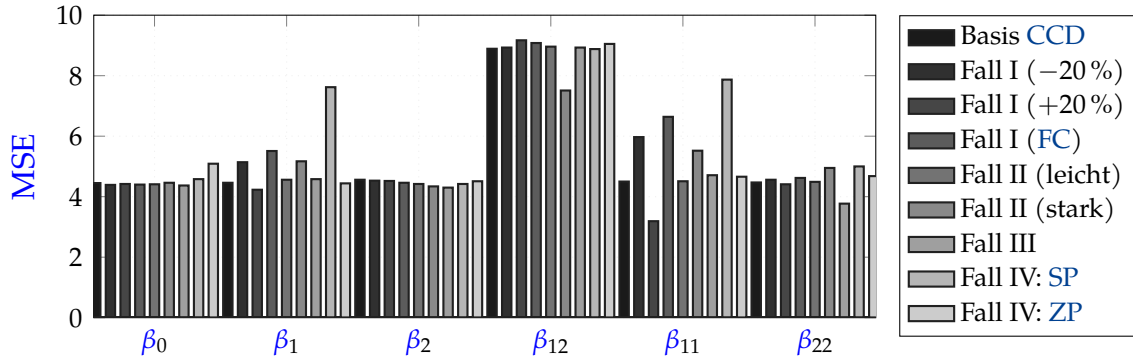
Abbildung C5: Güte der Schätzer (MSE) für \text{SNR} = 1 .
