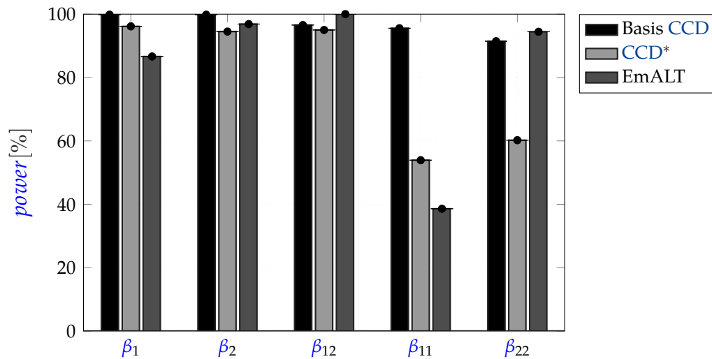
Abbildung 5.24: Absolutes Niveau der statistischen Trennschärfe ( power ) für das log-lineare Weibull-Modell. Das EmALT-Design sichert den wesentlichen quadratischen Term \hat{\beta}_{22} trotz Lebensdauerrauschen und asymmetrischer Restriktion mit nahezu 95 % verlässlich ab.
