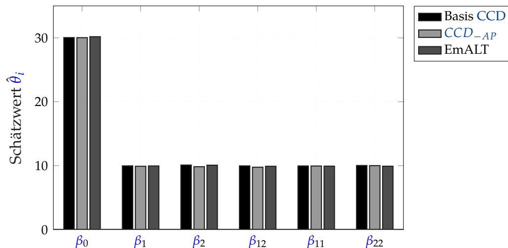
Abbildung 5.15: Absolute Schätzwerte der Modellkoeffizienten für die asymmetrischen Designvarianten am Arbeitspunkt \text{SNR} = 1,20 . Der Bias bleibt marginal; die Erwartungstreue des OLS-Schätzers bleibt gewahrt.
