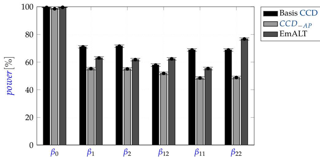
Abbildung 5.19: Vergleichende Analyse der statistischen Trennschärfe. Die asymmetrische Extrapolationsabsicherung (EmALT) stellt die Detektionsrate im Vergleich zur reinen Ausdünnung nahezu vollständig wieder her.
