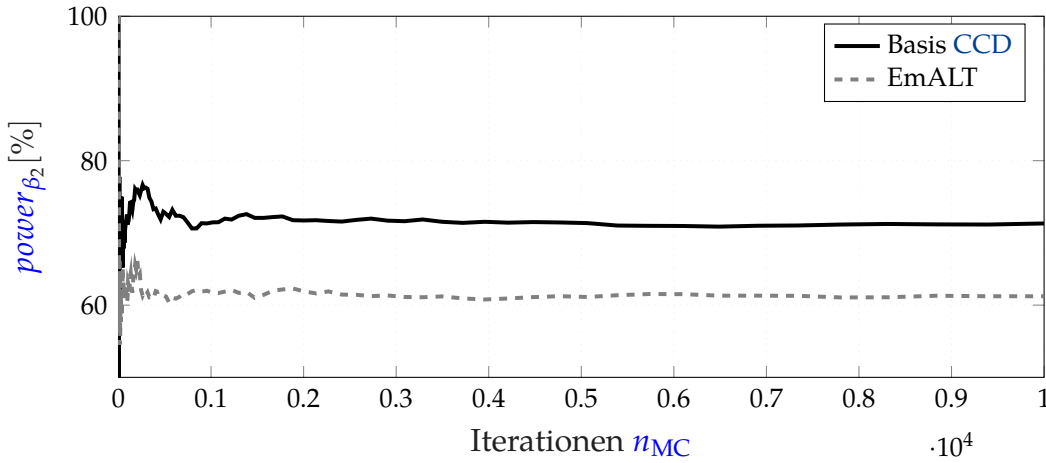
Abbildung 5.20: Numerische Konvergenz der empirischen Trennschärfe ( power ) über die Simulationsläufe.
