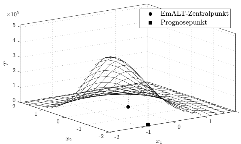
Abbildung 5.15: Antwortfläche der charakteristischen Systemlebensdauer T in Abhängigkeit der Faktoren x_1 und x_2 . Die Projektion verdeutlicht die massive Extrapolationsdistanz zwischen dem DoE-Zentrum und den geforderten Feld-Bedingungen.
