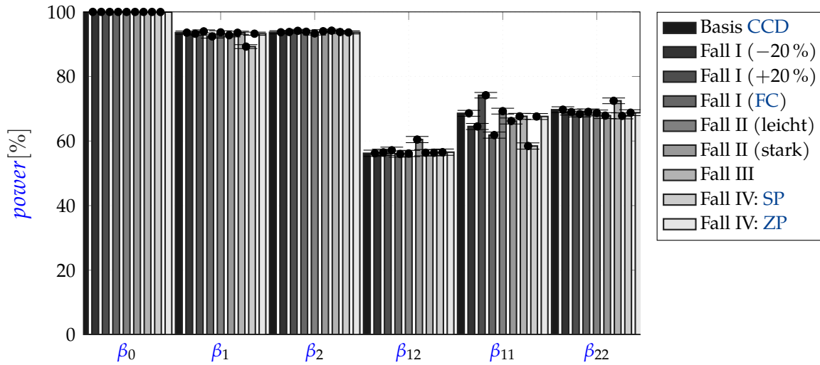
Abbildung 5.4: Trennschärfe mit 95 %-Konfidenzintervallen in Abhängigkeit der Störszenarien. Trotz kritischer Parameterkonstellation ( SNR = 1,20) bleiben die power -Verluste bei Erhalt der Symmetrie gering.
