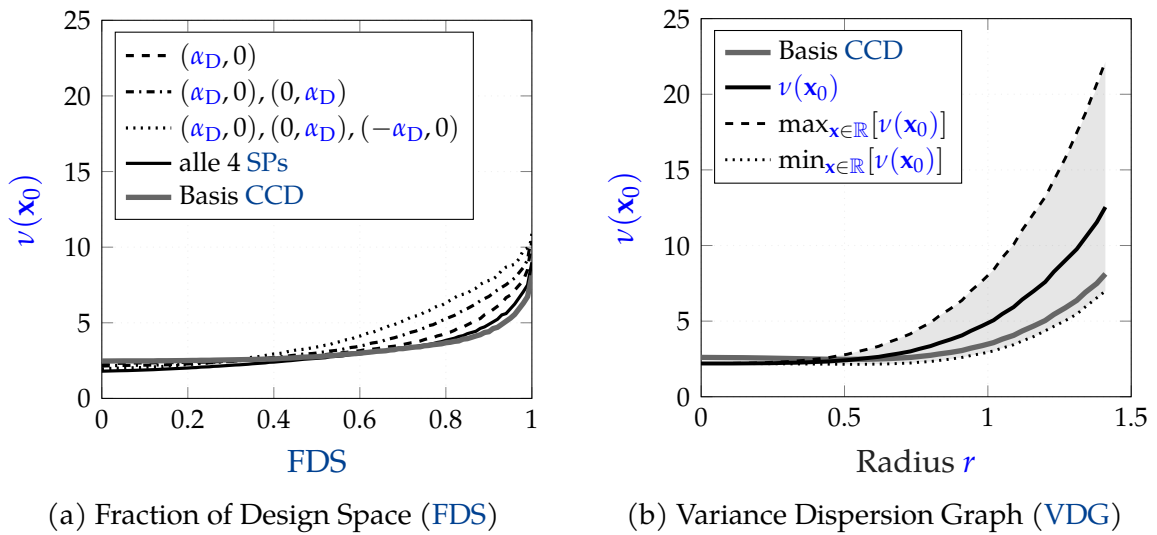
Abbildung 5.10: Vorhersagegüte bei Variation der SP -Anzahl n_{SP} für einen CCD mit k = 2 Faktoren. SPV -Werte für verschiedene Varianten entfallener Sternpunkte. Abbildung 5.10b zeigt den Fall des vollständigen Entfalls der Sternpunkte (\alpha_D; 0) und (0; \alpha_D) im Hochlastbereich.
