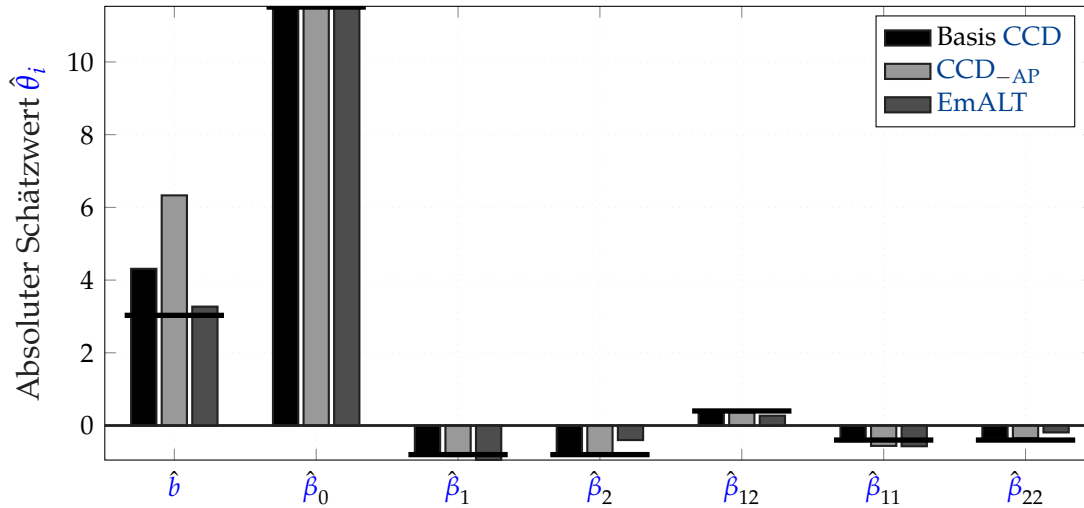
Abbildung 5.19: Absolute Schätzwerte der MLE-Koeffizienten im Weibull-Modell ( \text{SNR} = 1,20 ). Die Asymmetrie des EmALT provoziert keine unzulässigen systematischen Verzerrungen.
