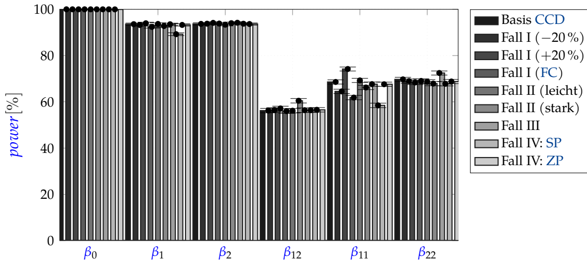
Abbildung 5.4: Trennschärfe mit 95 %-Konfidenzintervallen in Abhängigkeit der simulierten Störscenarien ( \text{SNR} = 1,20 ). Bei Erhalt der Basissymmetrie bleiben die power -Verluste bemerkenswert gering.
