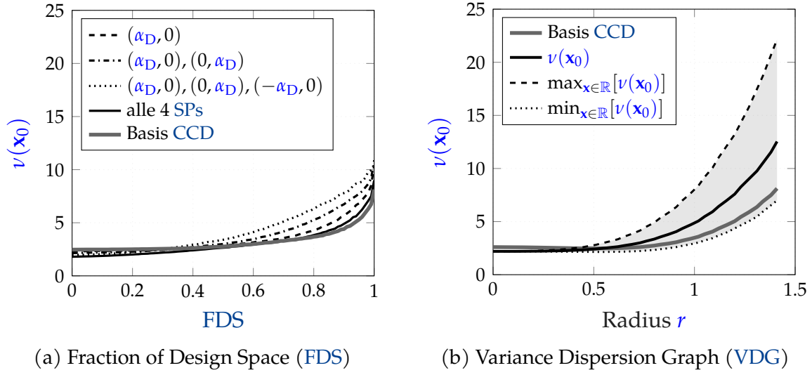
Abbildung 5.10: Vorhersagegüte bei Variation der SP-Anzahl n_{SP} für einen CCD mit k = 2 Faktoren. SPV-Werte für verschiedene Varianten entfallener Sternpunkte. Abbildung 5.10b zeigt den Fall des vollständigen Entfalls der Sternpunkte (\alpha_D; 0) und (0; \alpha_D) im Hochlastbereich.
