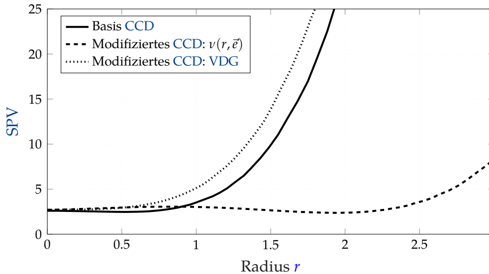
Abbildung 5.14: Der klassische VDG verschleiert den lokalen Design-Nutzen des um APs modifizierten CCD durch radiale Mittelung. Der EVG belegt hingegen die signifikante SPV-Reduktion zielgerichtet entlang des Extrapolationsvektors zum Prognosepunkt.
