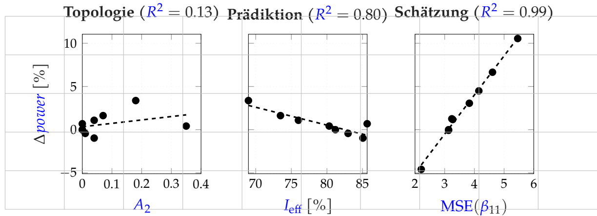
Abbildung 5.7: Korrelation zwischen a priori Design-Metriken und dem resultierenden Trennschärfe-Verlust in den Störszenarien: Der MSE übersetzt den geometrischen Fehler am direktesten in die probabilistische Trennschärfe.
