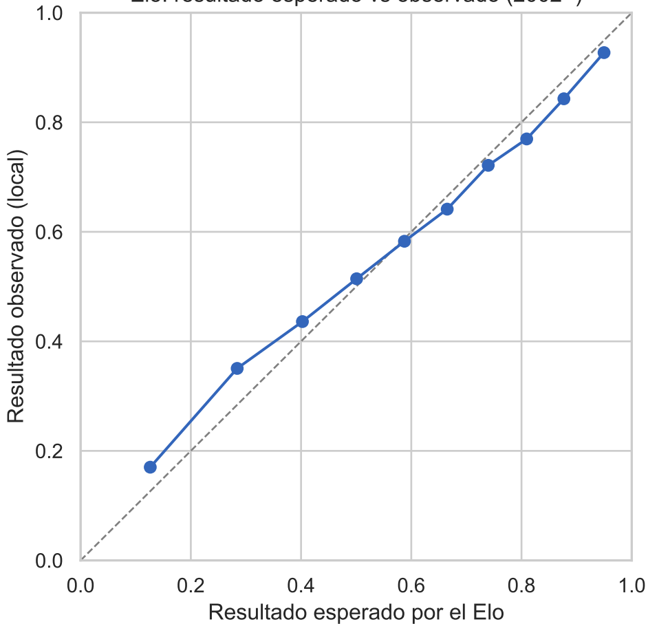
Elo: resultado esperado vs observado (2002+)
