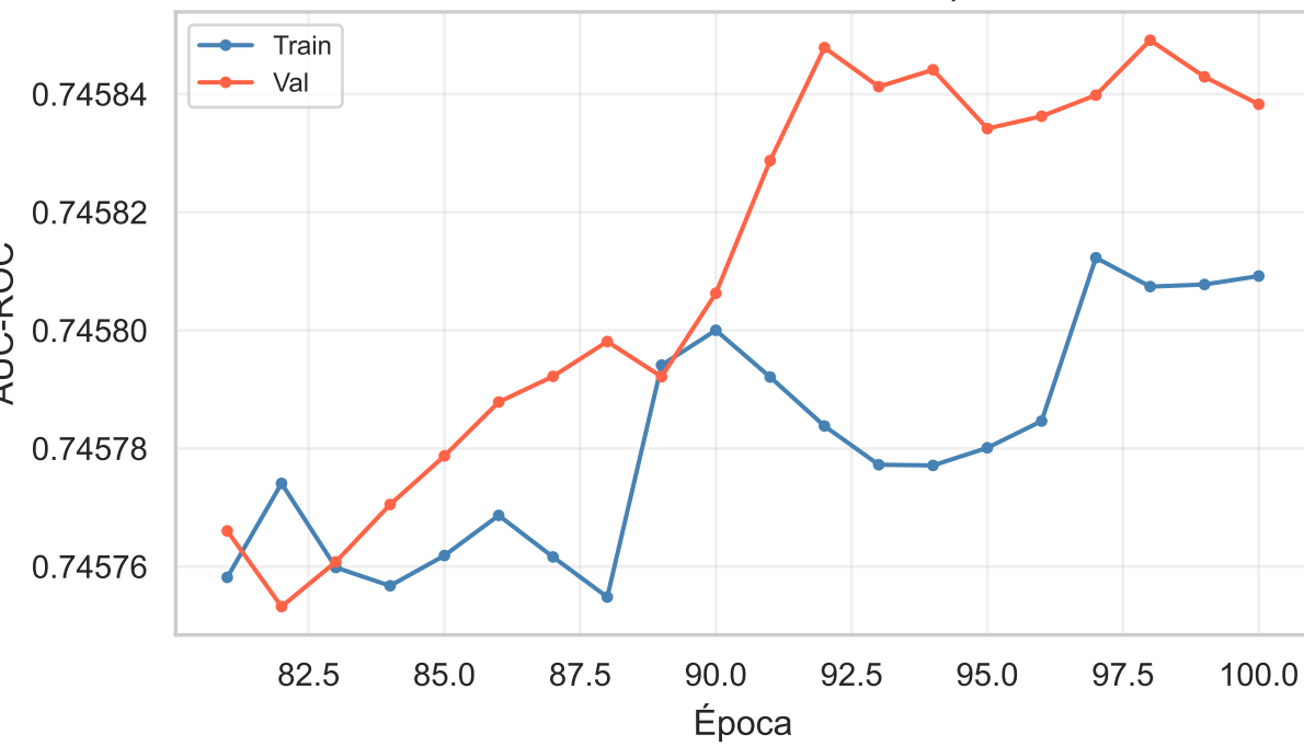
AUC-ROC — Zoom últimas 20 épocas
