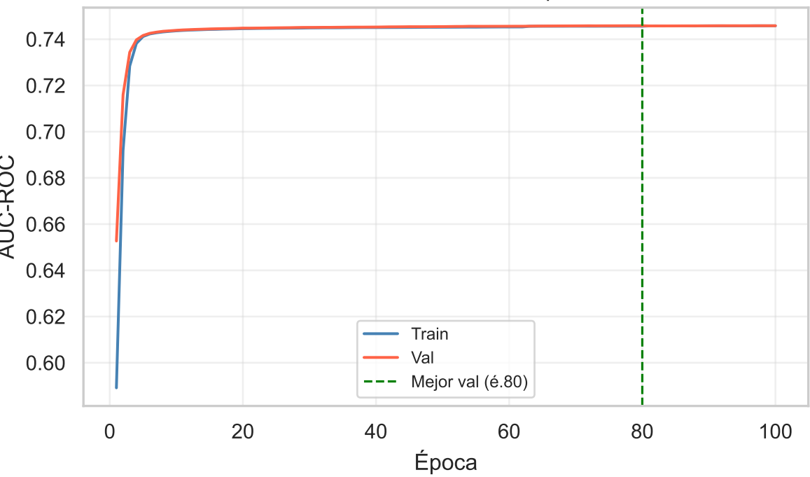
AUC-ROC — Curva completa
