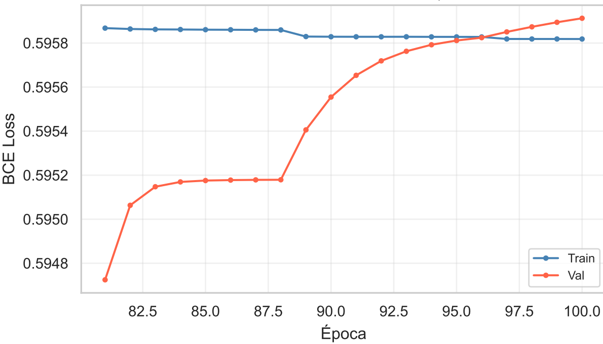
BCE Loss — Zoom últimas 20 épocas
