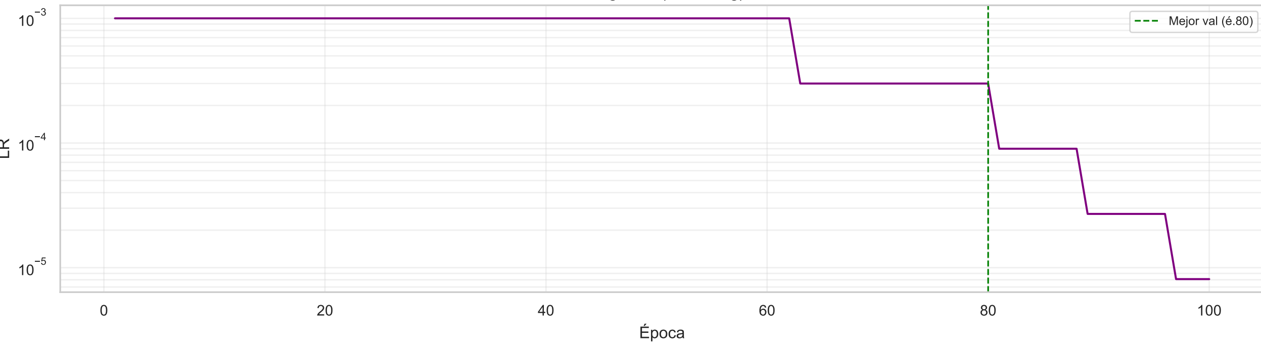
Evolución del Learning Rate (escala log) — 4 reducciones
