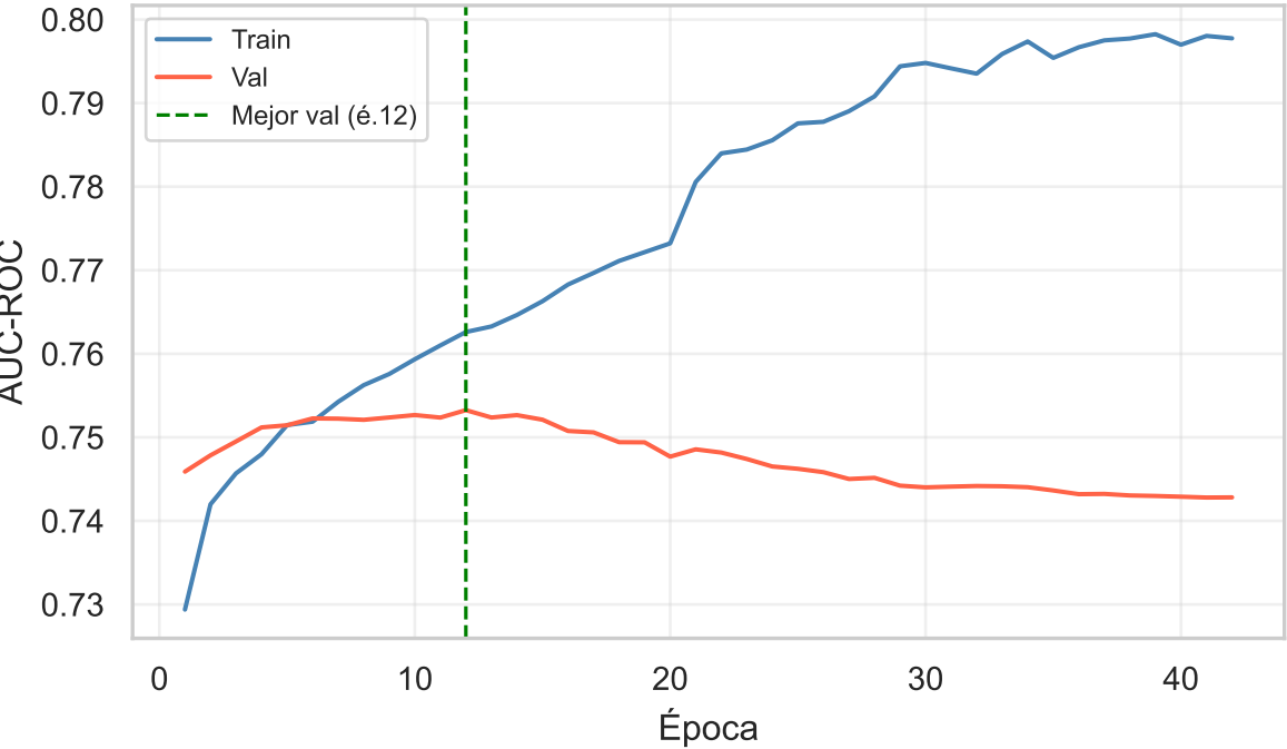
AUC-ROC — Curva completa
