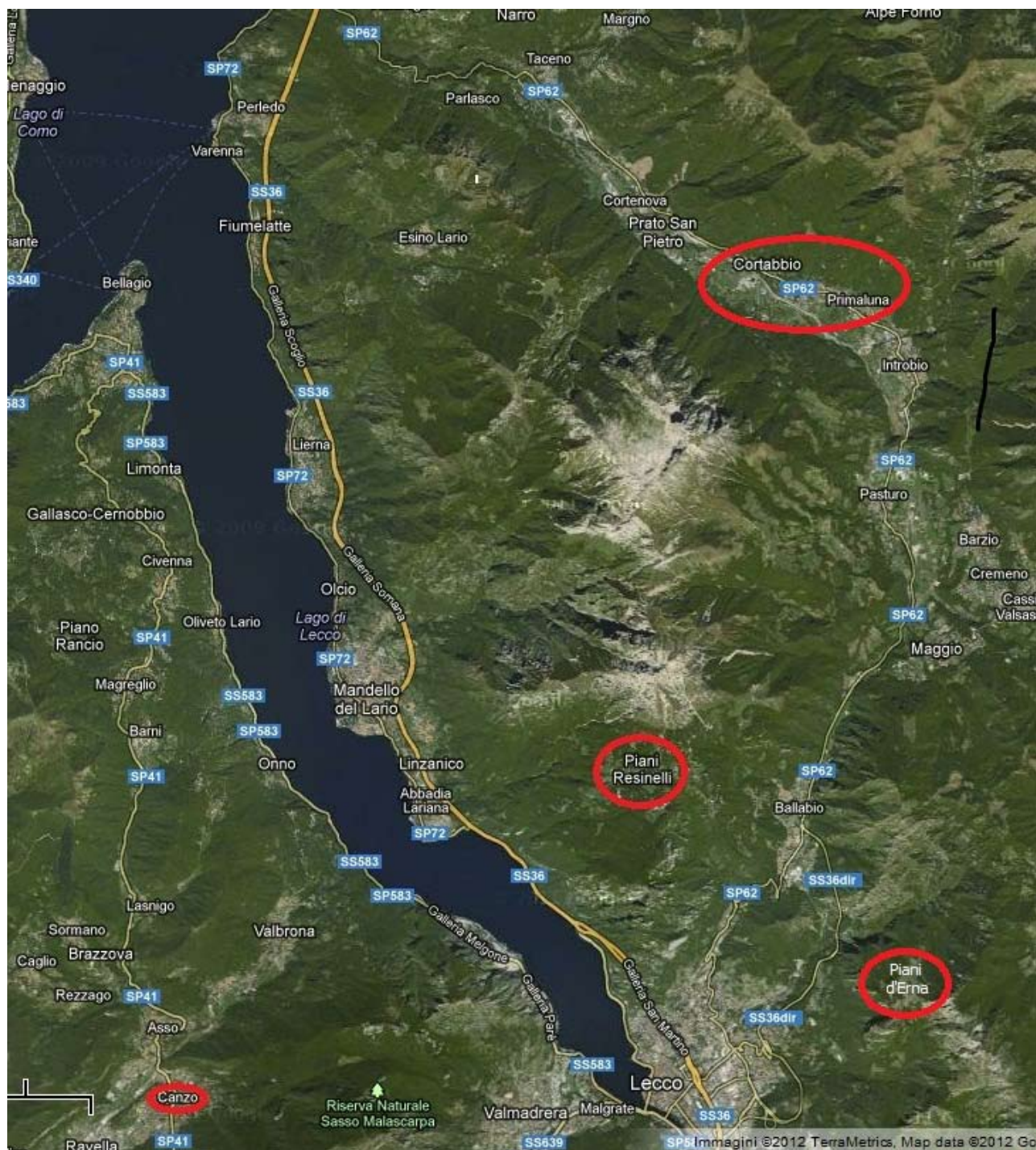
Fig. 1: Ubicazione delle zone minerarie della Lombardia occidentale citate nell'articolo (rielaborazione da Google Heart)
