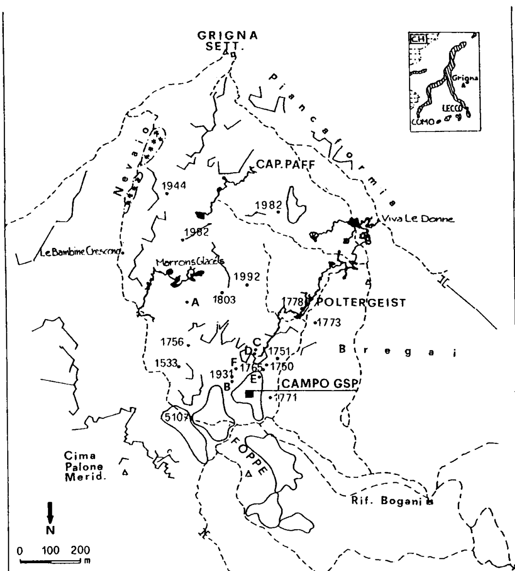
Da "Grotte e Abissi della Lombardia" (modif.)
