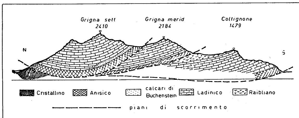
Fig. 1. — Sezione geologica Nord-Sud del gruppo delle Grigne (dai rilievi di De Sitter, Saibene e dati inediti di Gatti).
