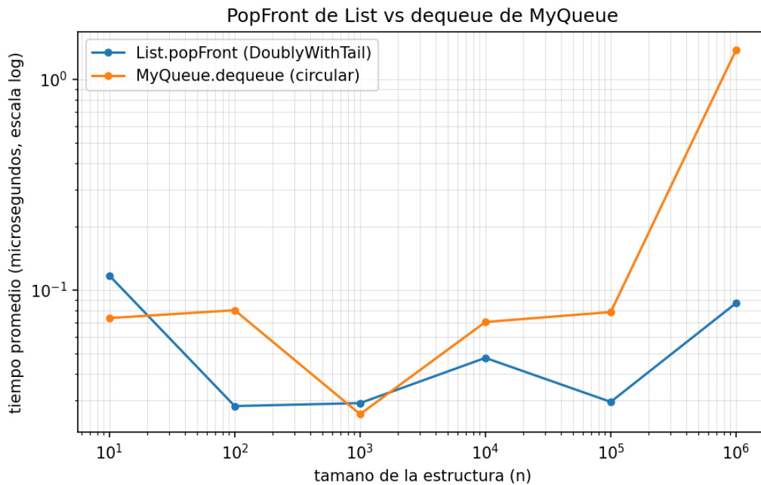
PopFront de List vs dequeue de MyQueue.
