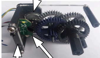
PCB para el sensado de velocidad
