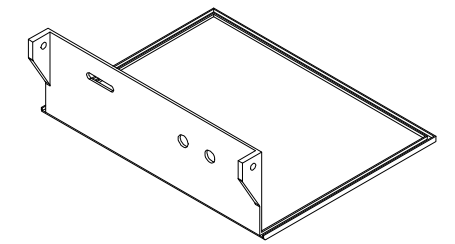
VISTA ISOMÉTRICA (ESCALA 1:5)
