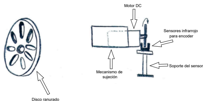
Figura 3.11.: Acople de encoder óptico
