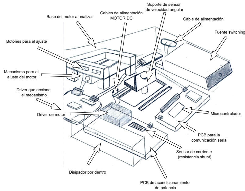
Figura 3.21.: Concepto 3 - Vista desde adentro del HW del sistema
