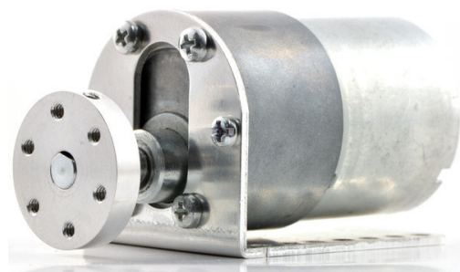
(b) Motor de la empresa Pololu utilizando el acople universal
