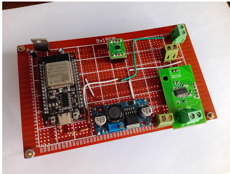
Figura 7.1.: Placa de pruebas diseñada para la implementación del prototipo.
