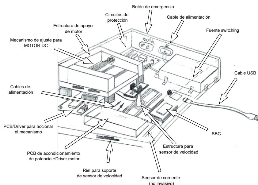
Figura 3.10.: Concepto 1 - Vista desde adentro del HW del sistema
