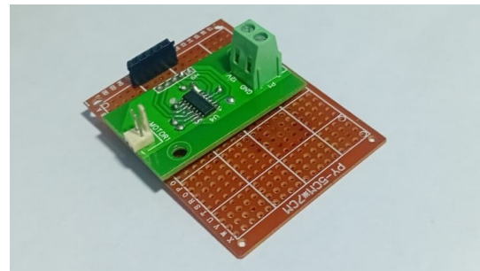
(b) Implementación física del driver VN7070BAS en una placa de pruebas.
