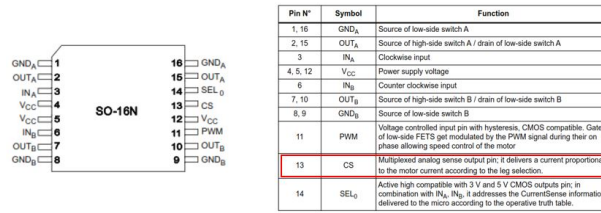
Figura 4.5.: Puente H VN7070BAS utilizado y salida de sensado de corriente (CS)
