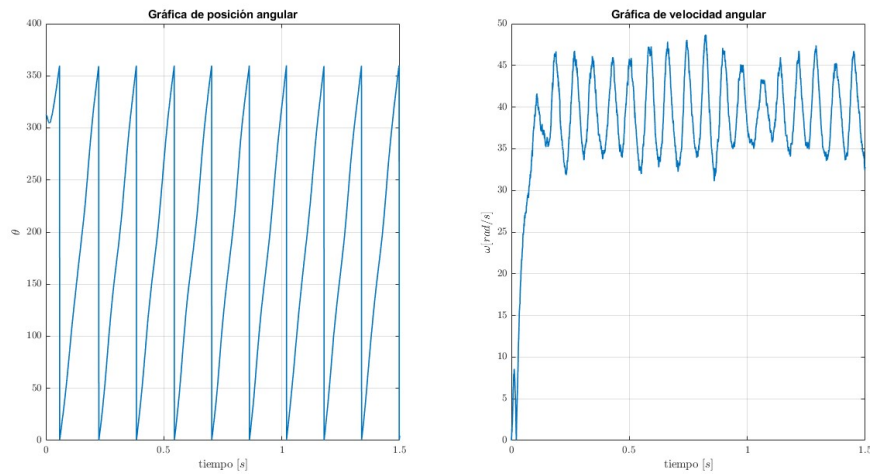
Figura 7.4.: Señales de posición angular y velocidad angular obtenidas a partir del TMAG5170A1.
