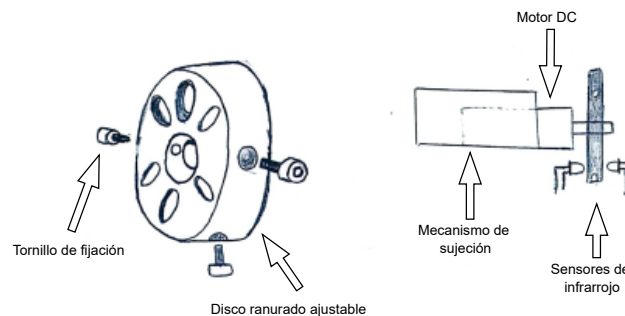
Figura 3.16.: Acople de encoder óptico ajustable a distintos diámetros de motor
