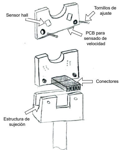
(a) Bosquejo de la tarjeta de sensado, tomando como referencia la Figura 3.19
