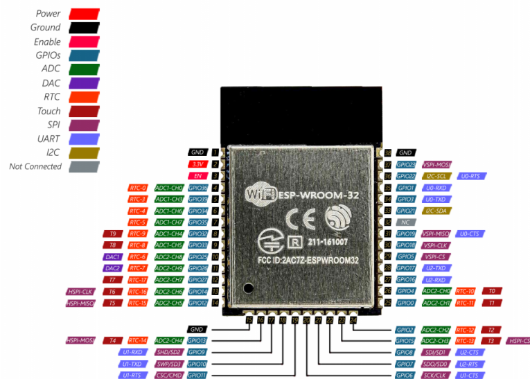
Figura 4.9.: Pinout del microcontrolador ESP32
