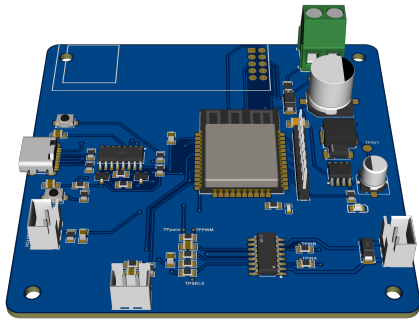
(a) Imagen referencial de cómo quedará la PCB de control
