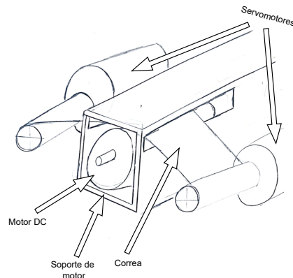
Figura 3.15.: Detalle de mecanismo de sujeción de motor DC para la solución 2
