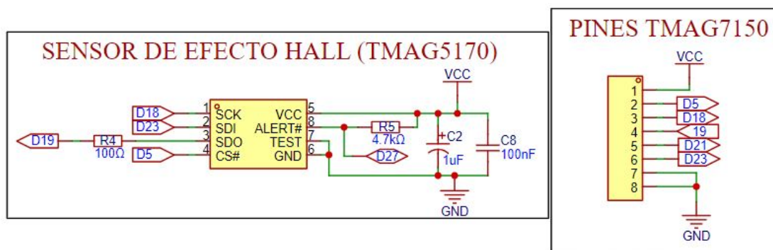
Figura 4.12.: Diagrama esquemático con las conexiones del sensor de efecto hall
