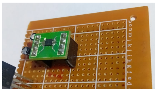
(b) Implementación de la PCB adaptadora para pruebas.
