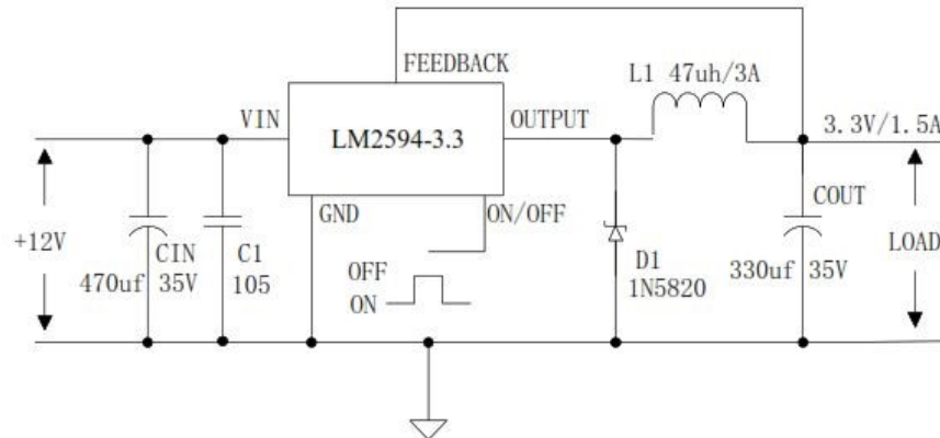
Figura 4.8.: Diseño típico de regulador LM2594
