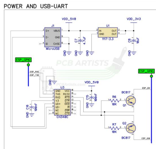
Figura 4.14.: Diagrama esquemático de referencia para diseñar el circuito de comunicación USB-UART
