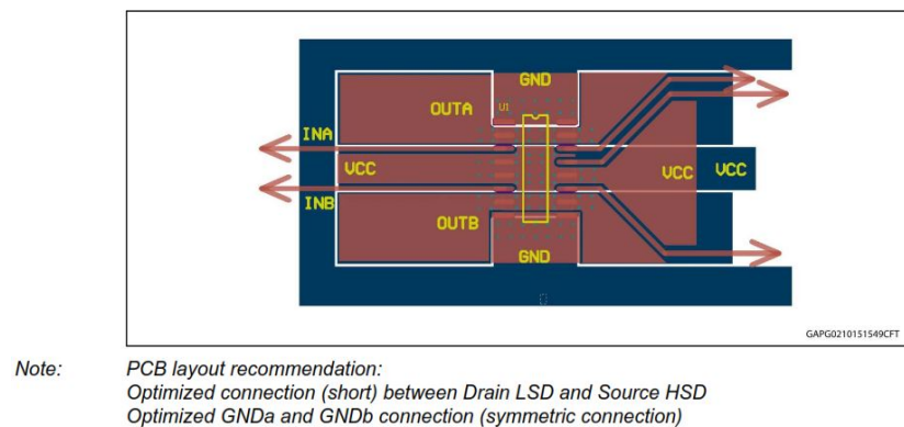
Figura 4.17.: Recomendación del fabricante respecto a las layers superficies de disipación y trazas del driver VN7070BAS
