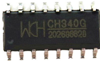
Figura 4.2.: Integrado CH340 cargar el programa y de poder comunicarse con el microcontrolador elegido
