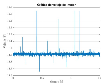
Figura 7.7.: Señal de voltaje de alimentación del motor obtenida durante las pruebas.
