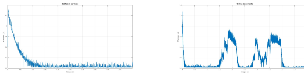
(a) Corriente durante el arranque del motor (1,5s). (b) Corriente con eje forzado durante un intervalo prolongado.
