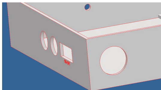
Figura 5.6.: Agujeros de la carcasa donde estarán los botones de Apagado, Encendido y de emergencia
