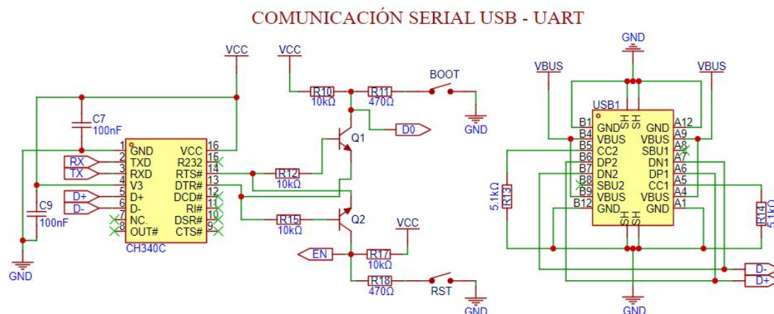
Figura 4.13.: Diagrama esquemático del circuito de comunicación USB-UART
