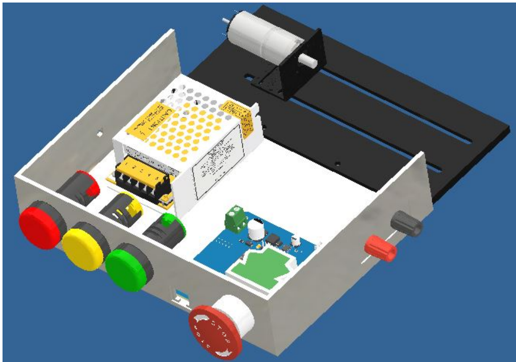
Figura 5.1.: Modelo CAD general del sistema mecánico del banco de pruebas.
