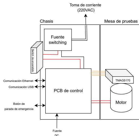
Figura 4.18.: Distribución de componentes y conectores (vista superior)
