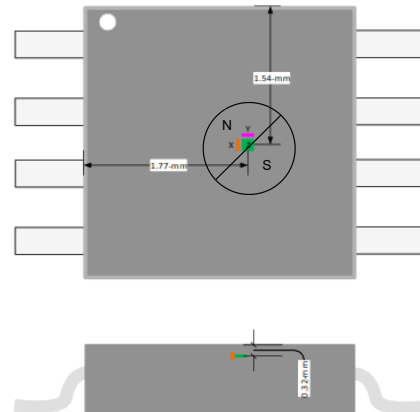
(b) Ubicación aproximada de la zona activa del sensor de efecto hall en el integrado.
