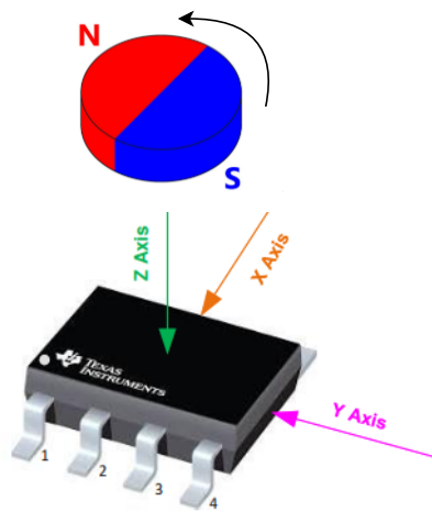
(a) Esquema de referencia para el montaje del imán respecto al sensor.
