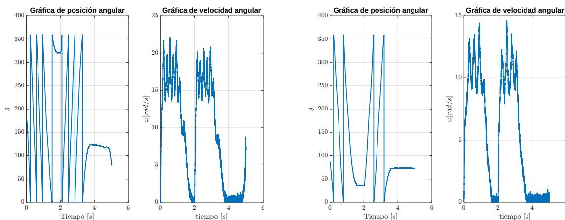
(a) Respuesta de velocidad angular del motor JGB37 ante señal de prueba.
