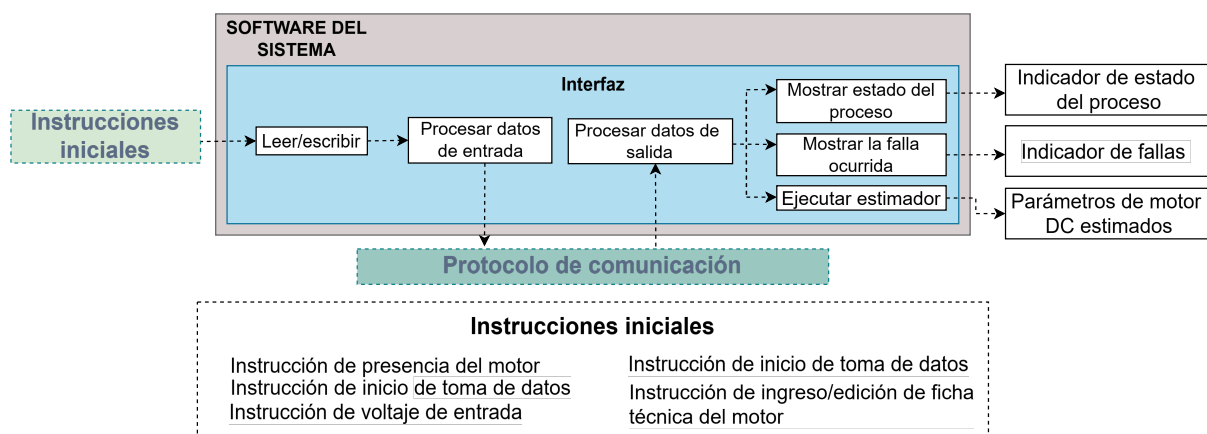
Figura 3.2.: Dominio de interfaz
