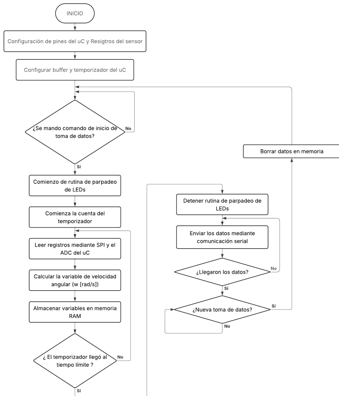
Figura 6.6.: Diagrama de flujo de la lógica de control utilizada para el sensado de variables.
