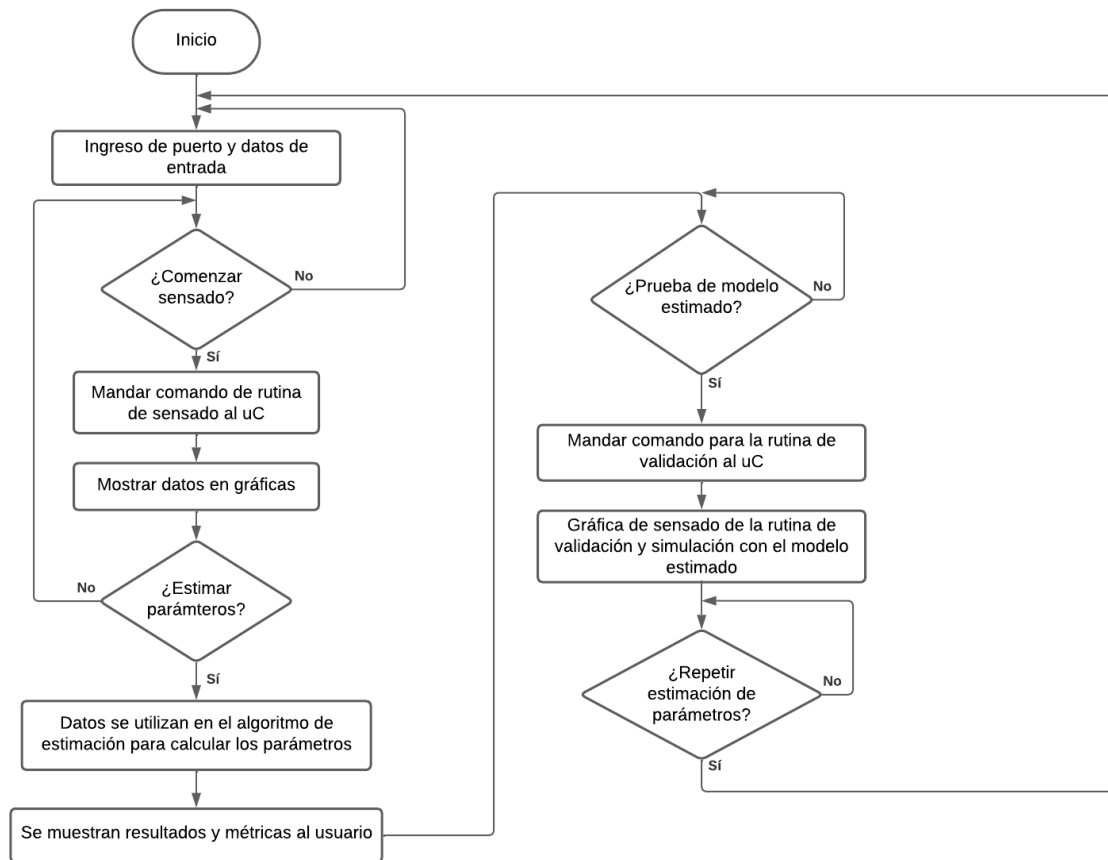
Figura 6.5.: Diagrama de flujo general de la lógica de la interfaz de usuario.
