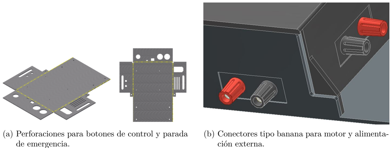
Figura 5.5.: Elementos principales de interfaz integrados en la carcasa.
