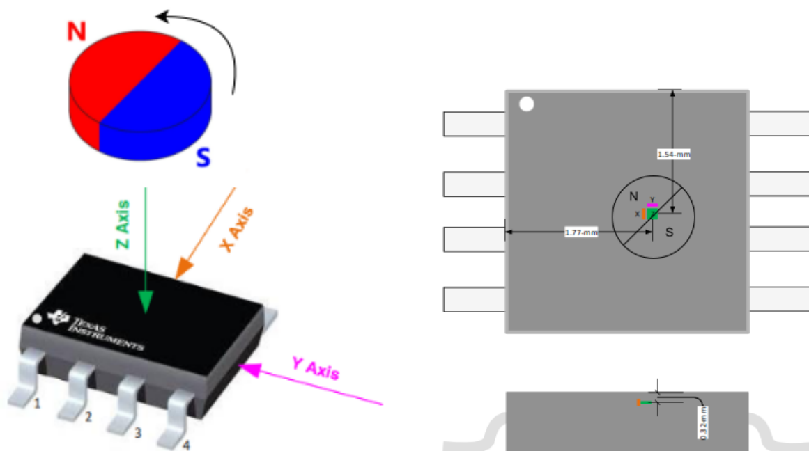
(a) Esquema de referencia para el montaje del imán respecto al sensor.
