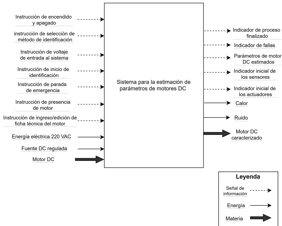
Figura 3.1.: Caja negra
