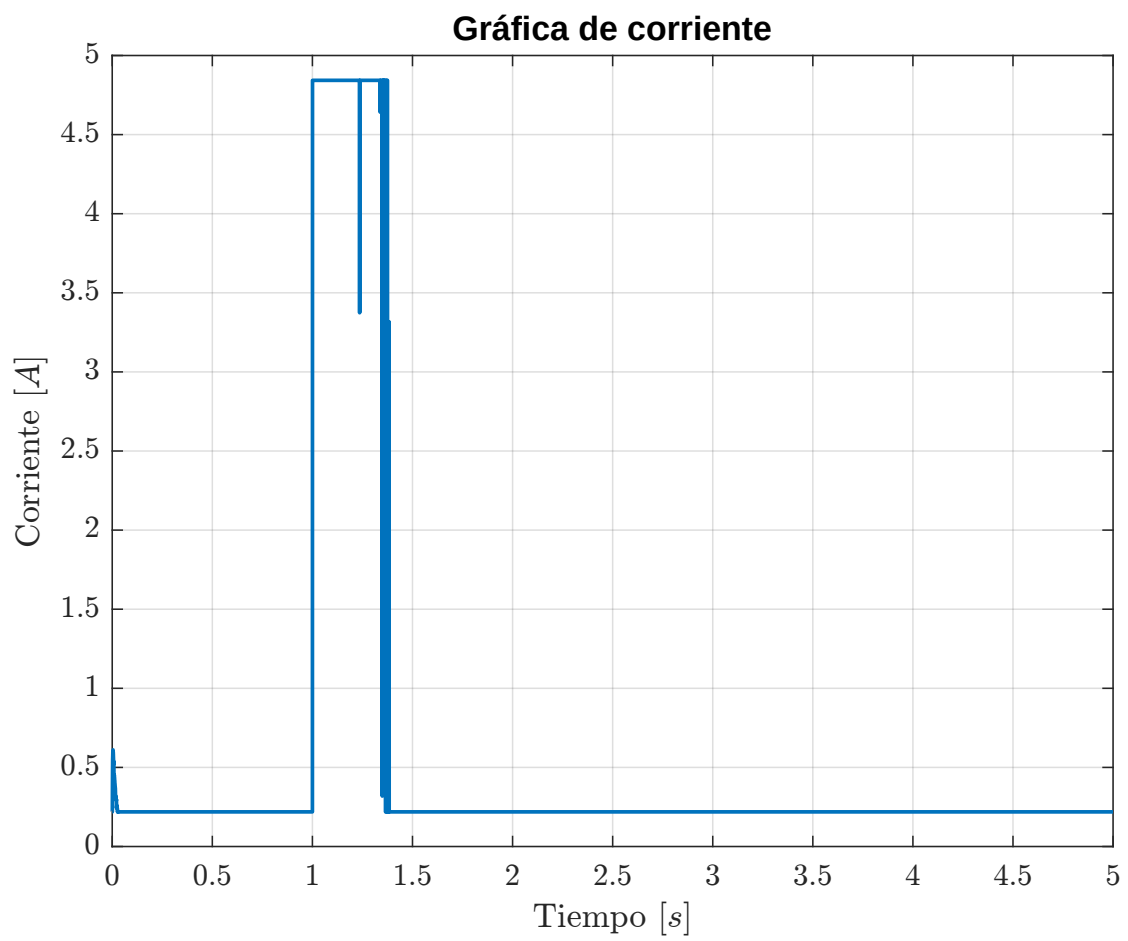
Figura 7.15.: Pico de corriente registrado al forzar la detención del motor.
