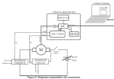
Figura 5. Diagrama esquemático de conexiones.
