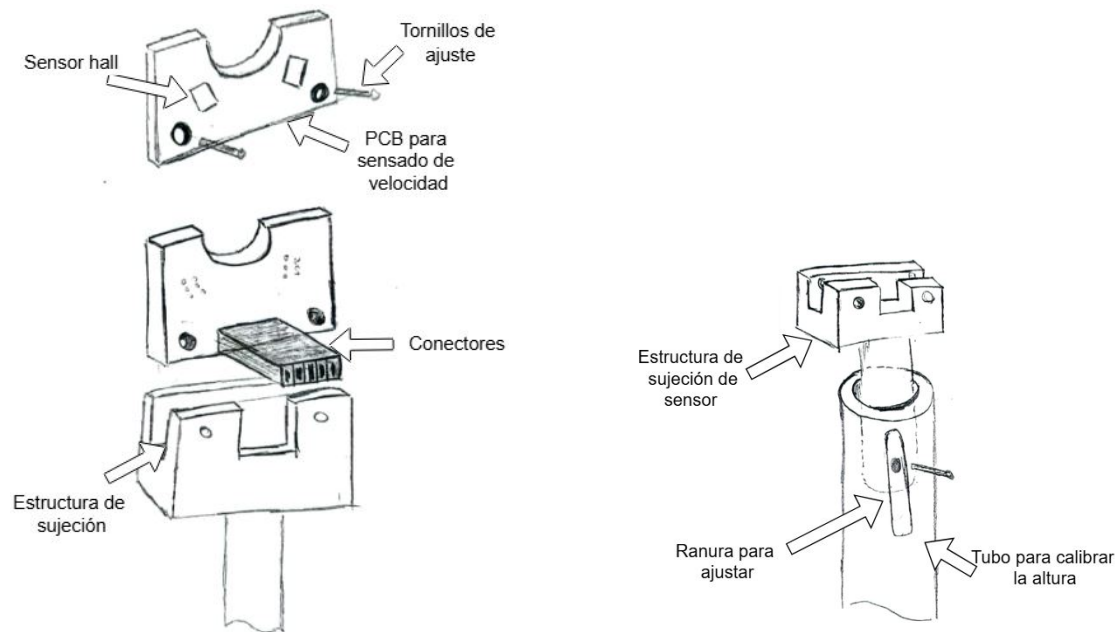
(a) Bosquejo de la tarjeta de sensado, tomando como referencia la Figura H.11
