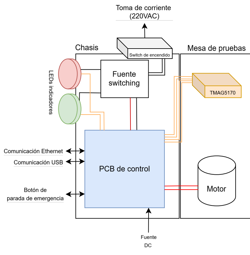
Figura 4.15.: Distribución de componentes y conectores (vista superior)
