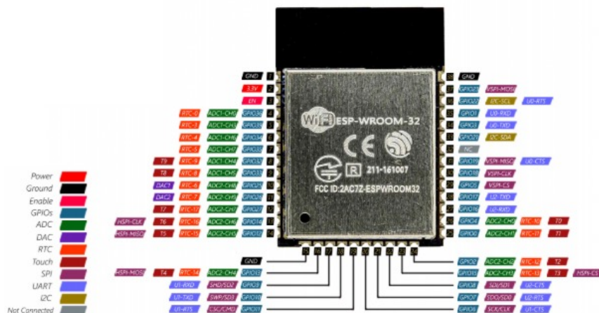
Figura 4.8.: Pinout del microcontrolador ESP32
