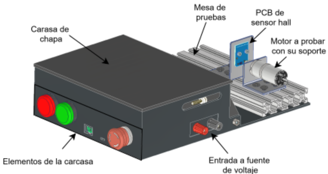
Figura 5.1.: Modelo CAD general del sistema mecánico del banco de pruebas.
