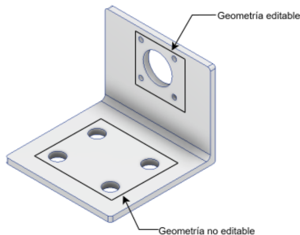
Figura 5.11.: Detalle referencial del bracket de motor
