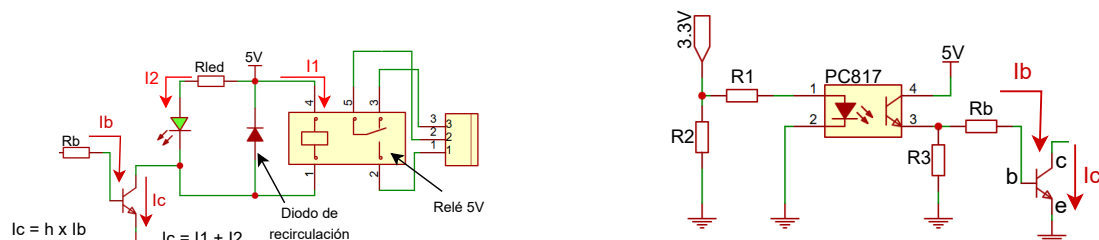
(a) Etapa de conmutación del relé mediante transistor 2N3904.
