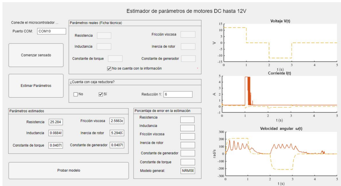
Figura 7.14.: Comparación entre la respuesta experimental y el modelo ideal construido con los parámetros estimados.
