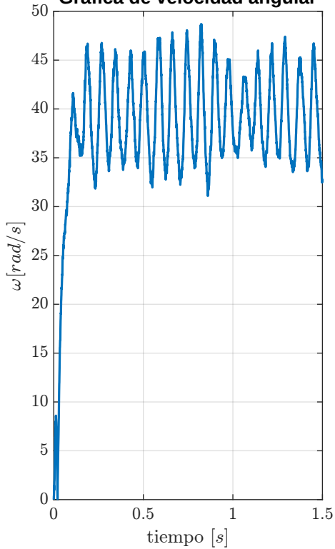
Gráfica de velocidad angular
