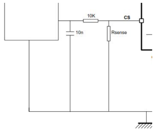
(a) Recomendación de implementación del sensado CS. (b) Tabla del factor de escalamiento típico de corriente.
