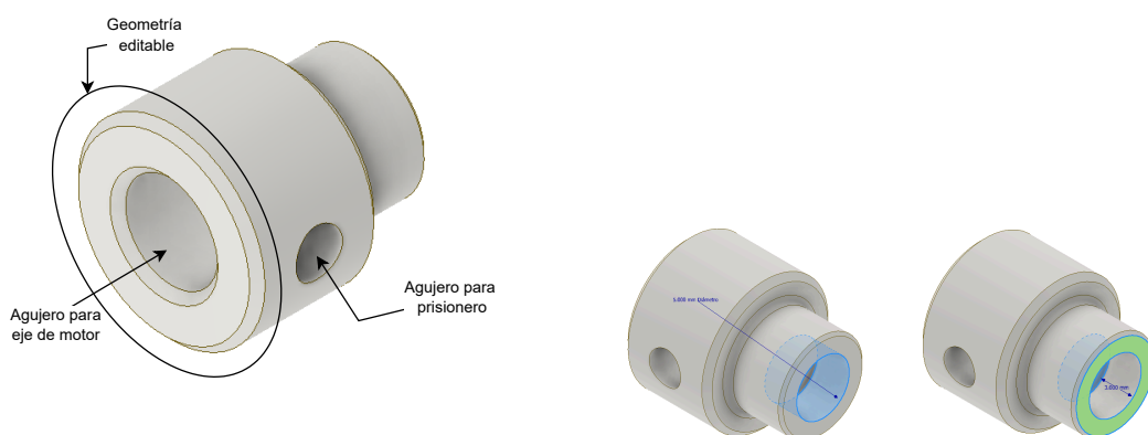
(a) Detalle general del acople: alojamiento del eje y orificio para prisionero (geometría editable según el eje). (b) Alojamiento del imán mediante inserción por presión (imán circular de 5 \times 3 mm).
