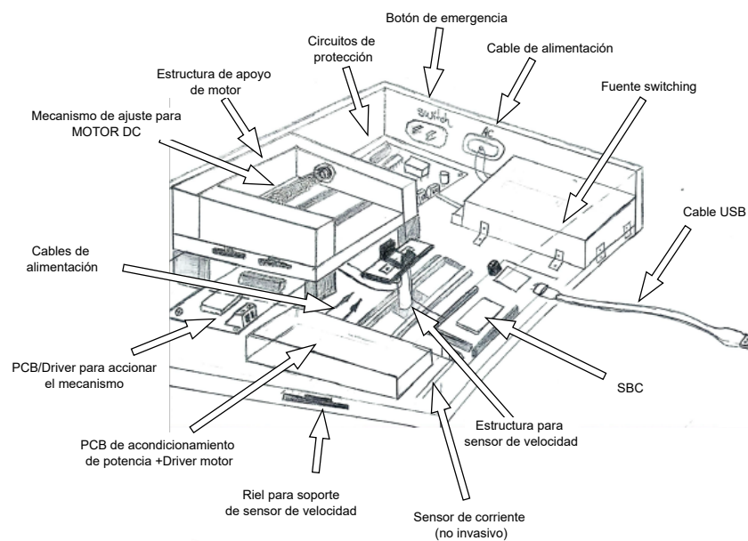
Figura H.2.: Concepto 1 - Vista desde adentro del HW del sistema
