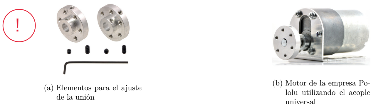
Figura 3.12.: Acople universal brindado por la empresa Pololu
