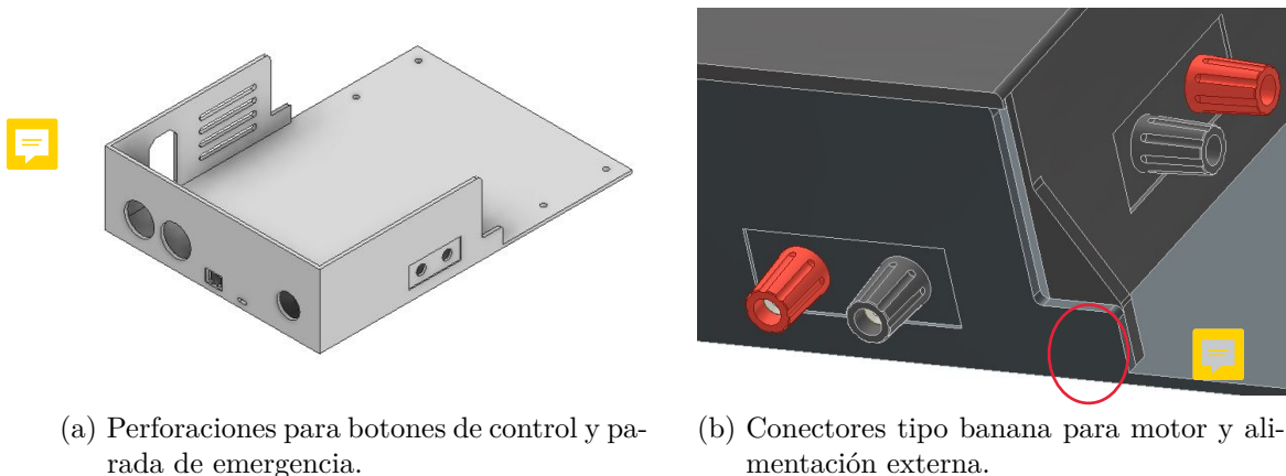
Figura 5.5.: Elementos principales de interfaz integrados en la carcasa.
