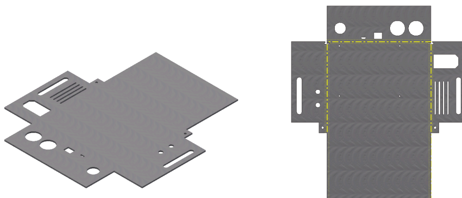
Figura 5.2.: Desarrollo de la plancha de chapa metálica (2 mm, 364 \times 330 mm) con recortes, perforaciones y líneas de doblez para el chasis.
