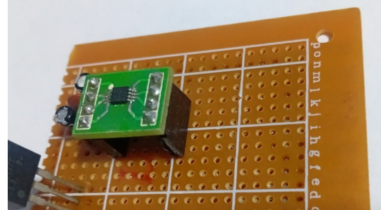
(b) Implementación de la PCB para pruebas.
