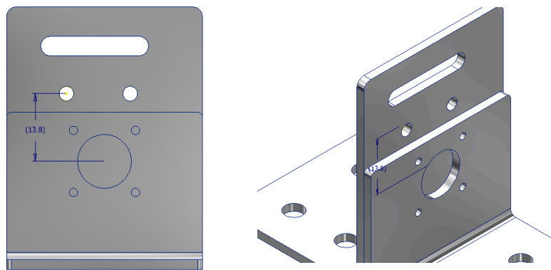
Figura 5.15.: Referencia de separación centro–centro entre el bracket del motor y el bracket del sensor para asegurar la coaxialidad.
