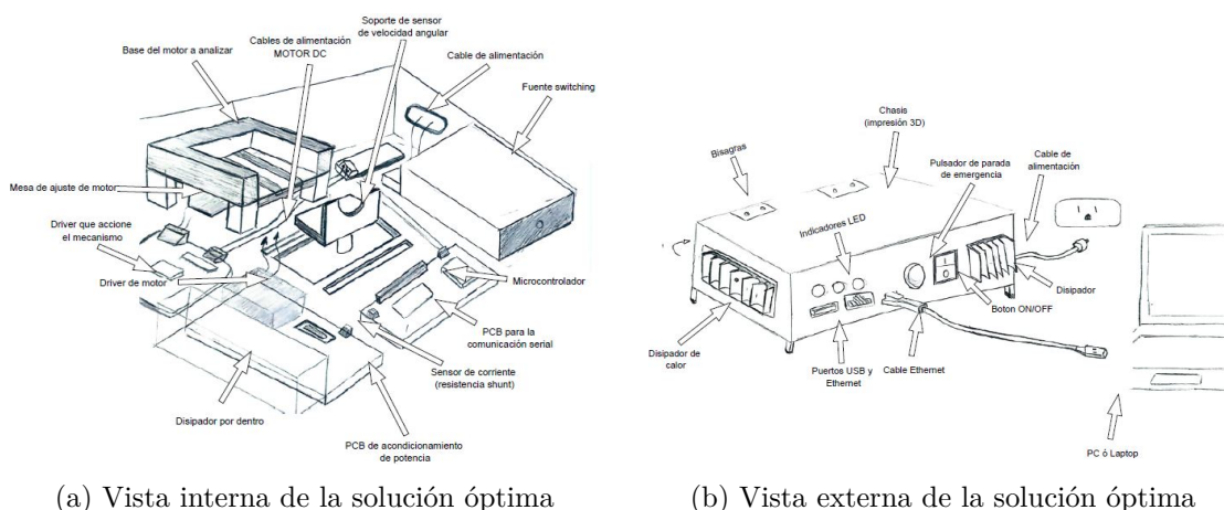
Figura 3.9.: Vistas interna y externa de la solución óptima seleccionada.
