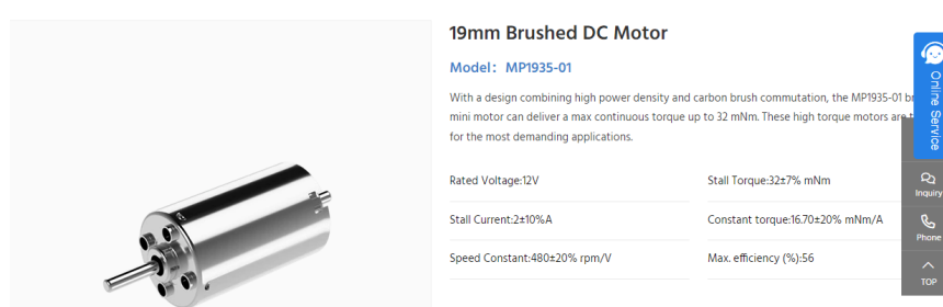
Figura 2.4.: Imagen referencial del motor cotizado en la página de Zhaowei
