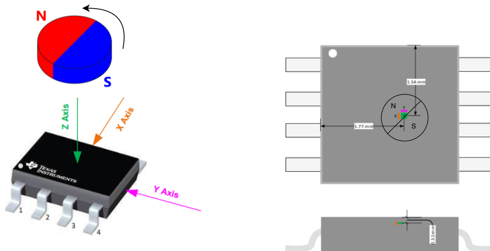
(a) Esquema de referencia para el montaje del imán respecto al sensor.
