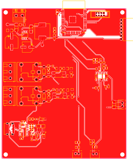
(a) Layer Top de la tarjeta de control.
