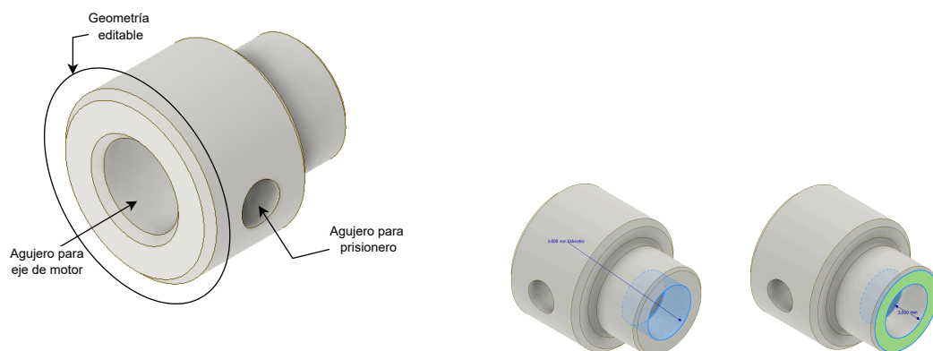
(a) Detalle general del acople: alojamiento del eje y orificio para prisionero (geometría editable según el eje). (b) Alojamiento del imán mediante inserción por presión (imán circular de 5 \times 3 mm).
