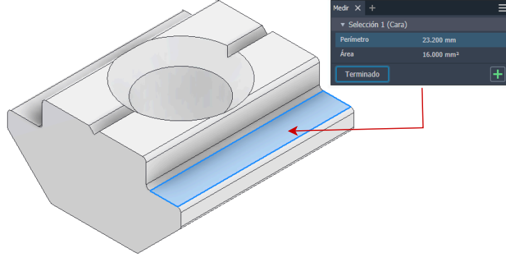
Figura 5.9.: Área de contacto referencial entre la tuerca tipo martillo y el perfil V-SLOT.
