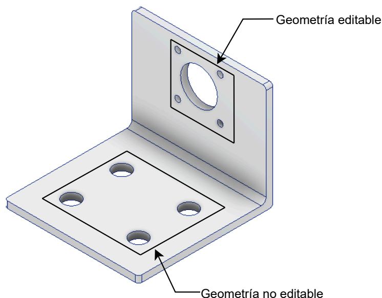
Figura 5.11.: Detalle referencial del bracket de motor
