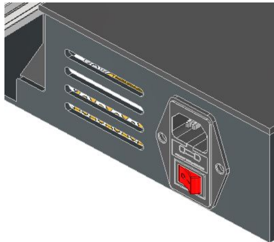
Figura 5.7.: Interruptor general con fusible integrado para corte y protección al inicio de la alimentación.
