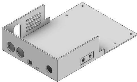
(a) Perforaciones para botones de control y parada de emergencia.
