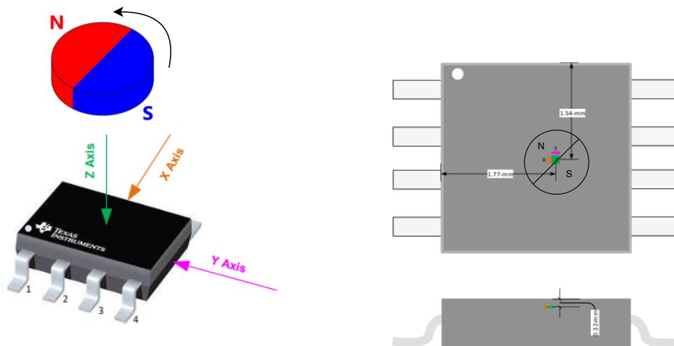
(a) Esquema de referencia para el montaje del imán respecto al sensor. (b) Ubicación aproximada de la zona activa del sensor de efecto hall en el integrado.
