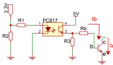
(a) Etapa de conmutación del relé mediante transistor 2N3904. (b) Etapa de aislamiento mediante optoacoplador PC817.
