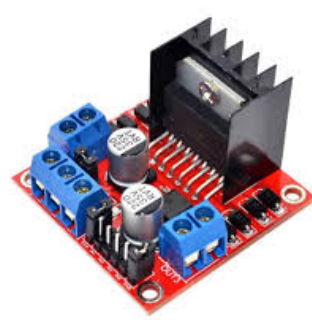
(b) L298N
