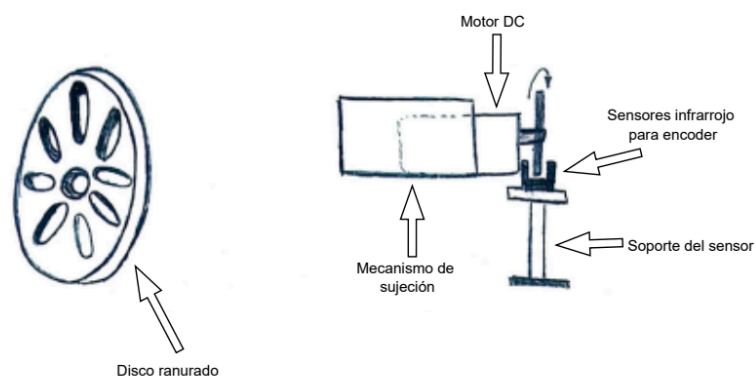
Figura 3.11.: Acople de encoder óptico
