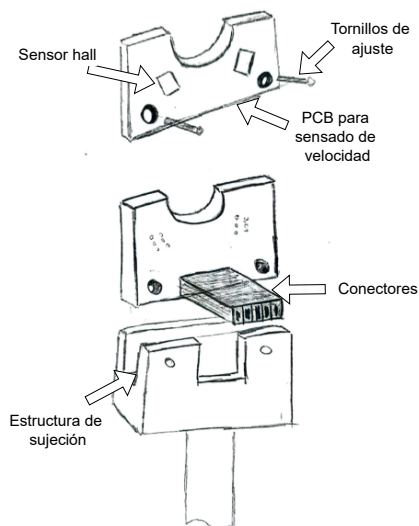
(a) Bosquejo de la tarjeta de sensado, tomando como referencia la Figura 3.19
