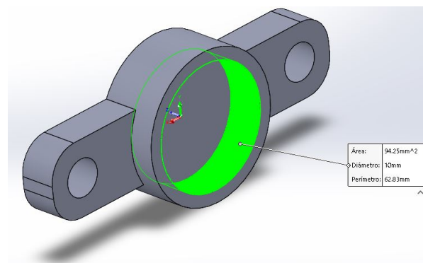
Figura 5.3.: Bujes de fijación para motores de la marca pololu
