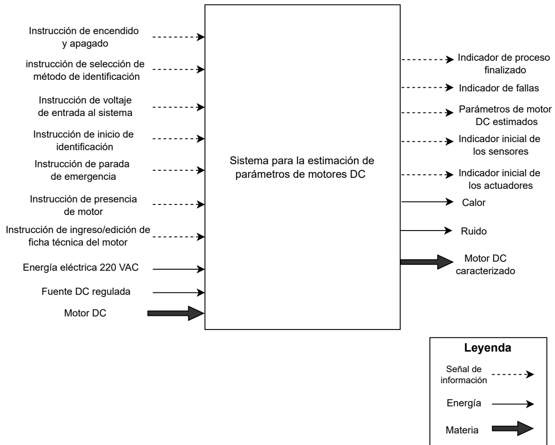
Figura 3.1.: Caja negra
