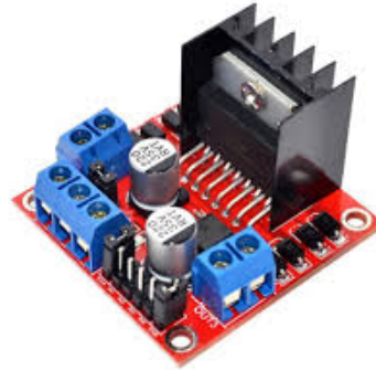
(b) L298N
