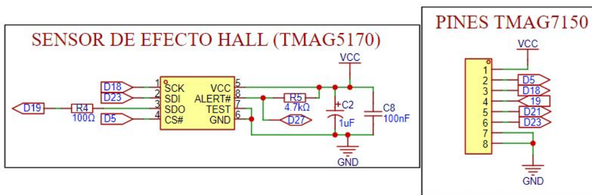
Figura 4.12.: Diagrama esquemático con las conexiones del sensor de efecto hall
