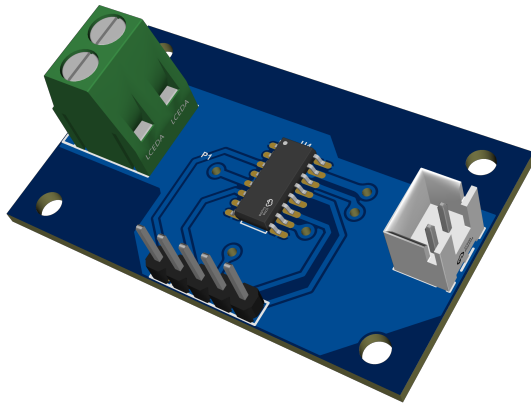
(a) Diseño de la PCB del driver VNH7070BAS en EasyEDA
