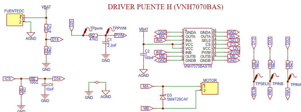
Figura 4.11.: Diagrama esquemático de conexiones con el driver VNH7070BAS
