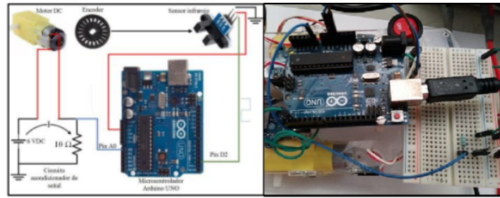
Figura 2.6.: Implementación experimental para la toma de datos
