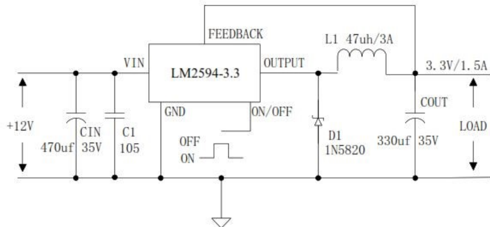
Figura 4.8.: Diseño típico de regulador LM2594
