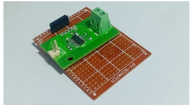
(b) Implementación física del driver VNH7070BAS en una placa de pruebas
