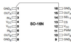
Figura 4.5.: Puente H VN7070BAS utilizado y salida de sensado de corriente (CS)
