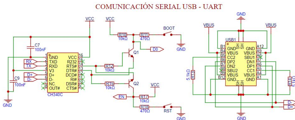
Figura 4.13.: Diagrama esquemático del circuito de comunicación USB-UART
