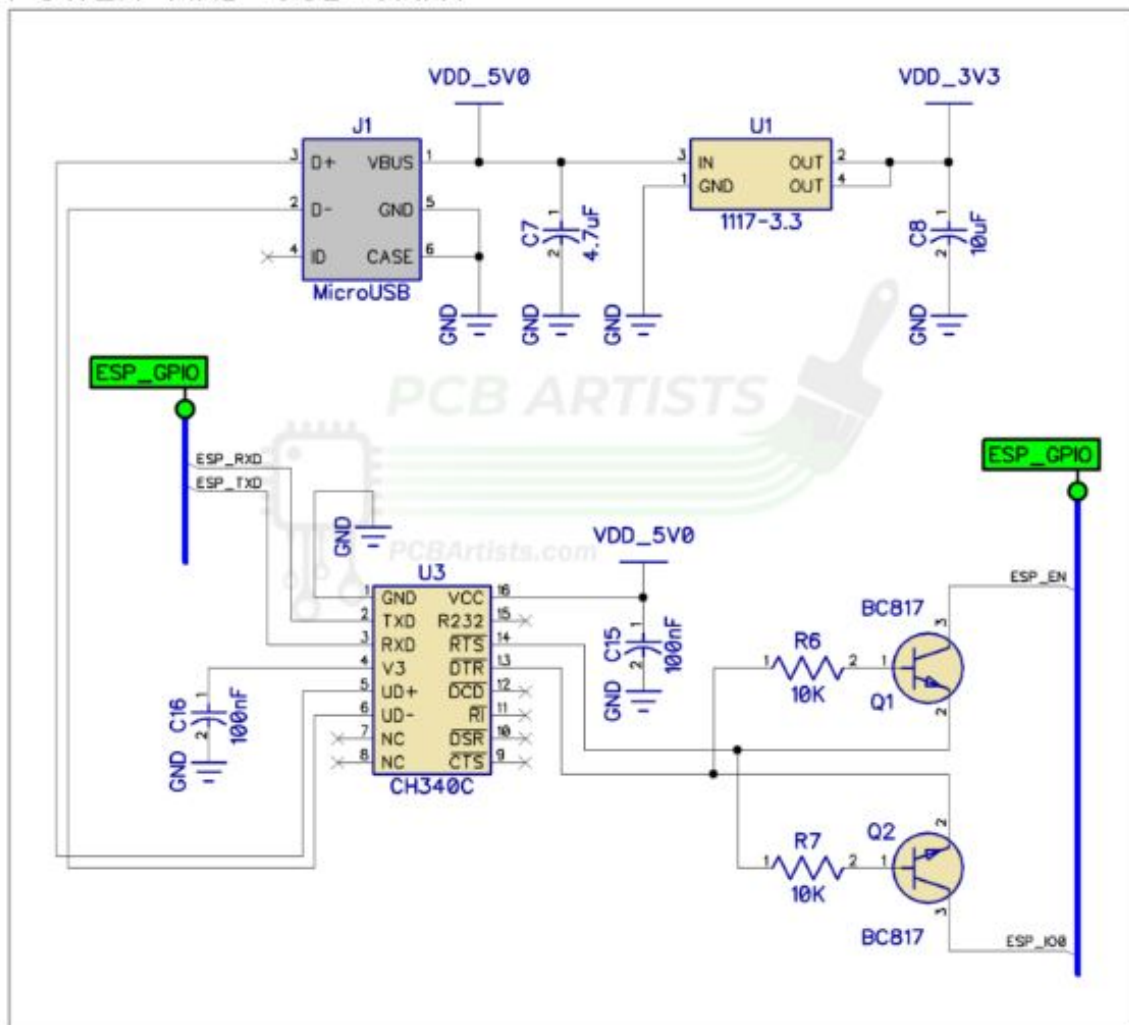
Figura 4.14.: Diagrama esquemático de referencia para diseñar el circuito de comunicación USB-UART
