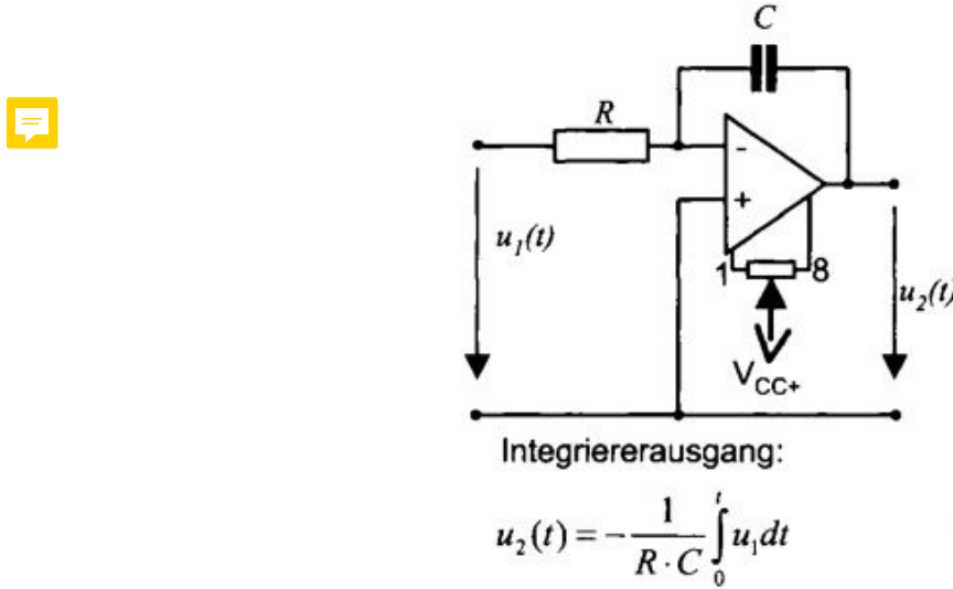
Figura C.4.: Circuito de un amplificador integrador realiza la función matemática de la integración de la señal de entrada. Extraído de (Scherf, 2008)
