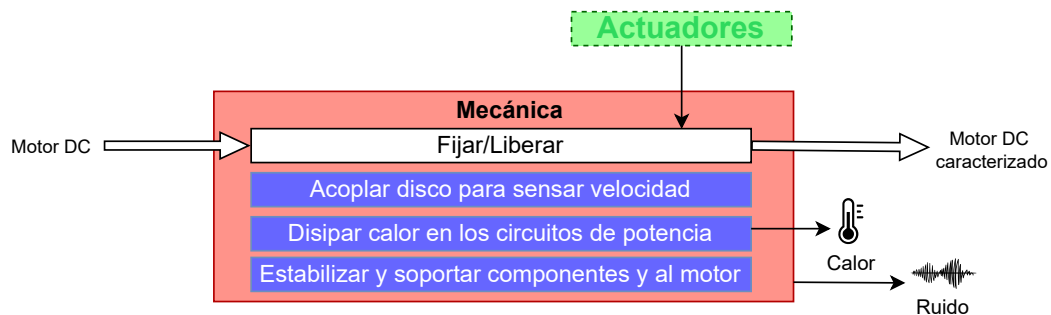
Figura 3.7.: Dominio mecánico
