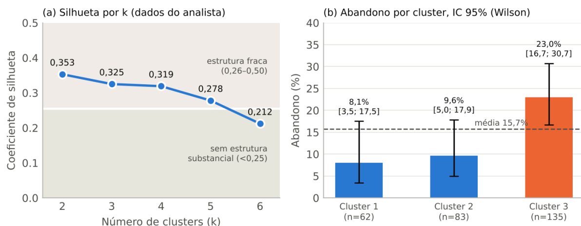
Figura A. (a) Silhueta por k com as faixas de Kaufman e Rousseeuw (1990). (b) Abandono por cluster com IC a 95% (Wilson), reconstruído a partir de n × taxa.
