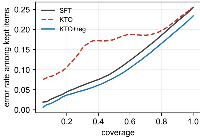
LFM2.5-1.2B
