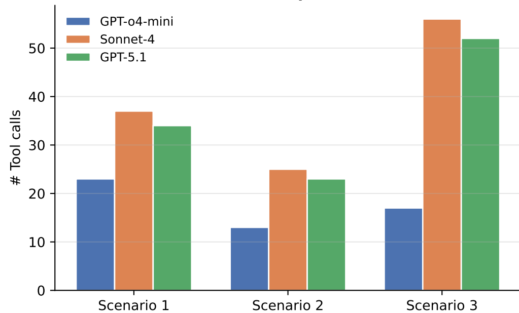
MCP Tool Calls per Scenario
