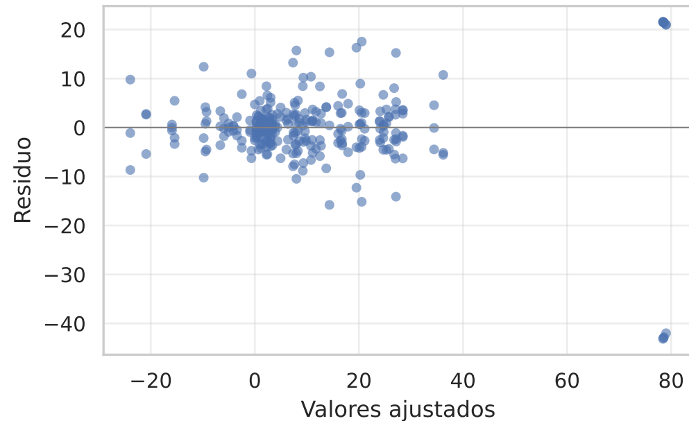
Residuos vs ajustados
