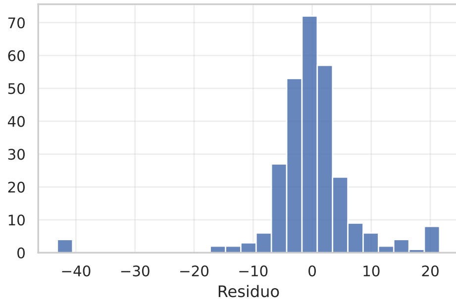
Histograma de residuos
