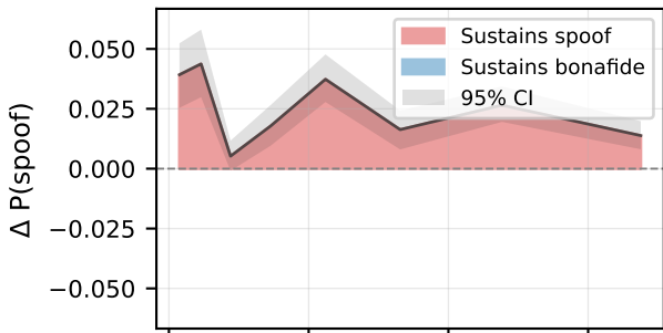
D_{zs} (zero-shot)
