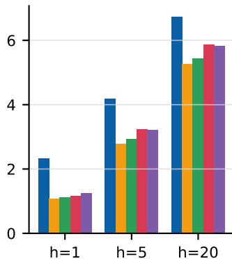
MAE
