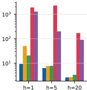
QLIKE (log scale)
