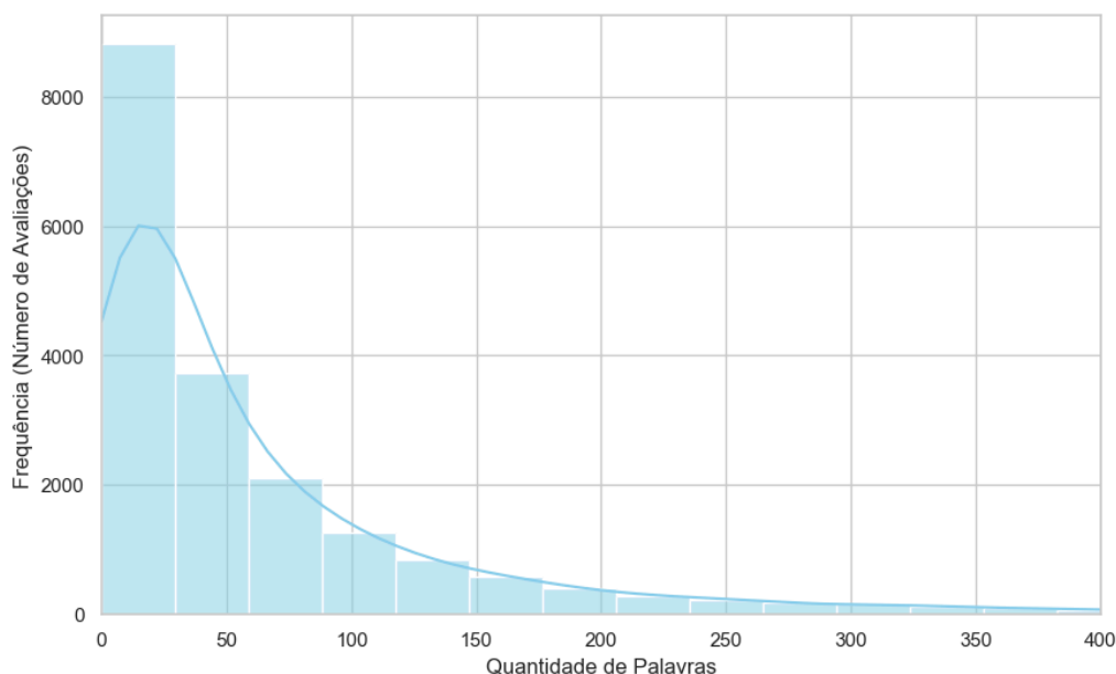
Figura 1: Distribuição da quantidade de palavras nas avaliações textuais
