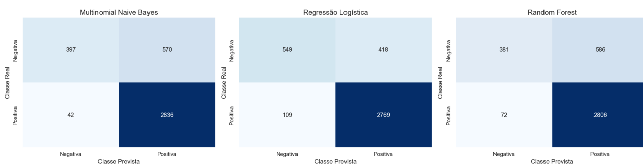
Figura 3: Matrizes de Confusão dos Modelos Avaliados
