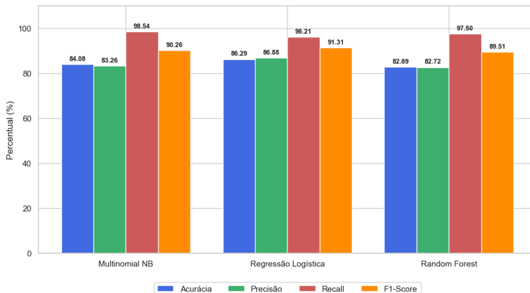
Figura 4: Comparação de Desempenho dos Modelos
