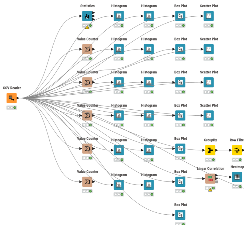
Figura A.1: Workflow da fase de Compreensão dos Dados no KNIME
