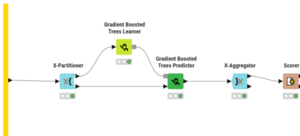
Figura 27: Metanódo do modelo Gradient Boosted Trees no KNIME
