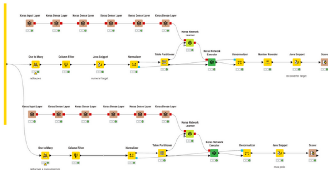
Figura 29: Metanode do modelo Keras no KNIME
