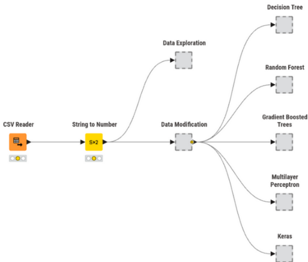
Figura 22: Visão geral do workflow desenvolvido no KNIME para o dataset atribuído
