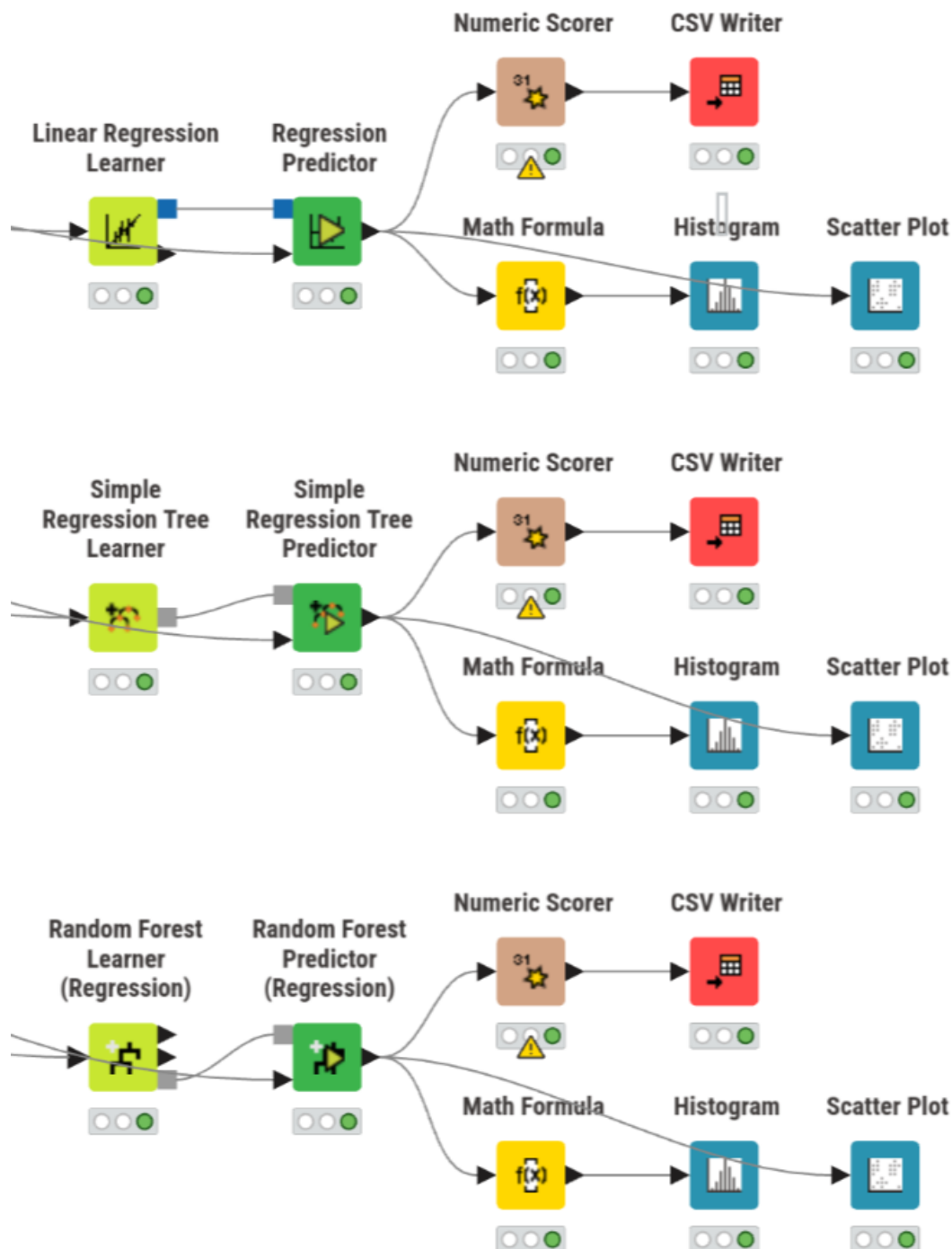
Figura 18: Workflow da fase de Regressão no KNIME
