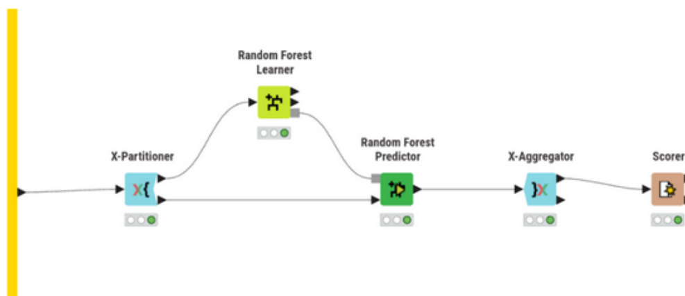
Figura 26: Metanode do modelo Random Forest no KNIME
