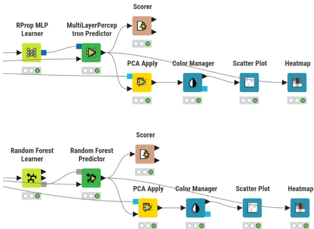
Figura 14: Workflow da fase de Classificação no KNIME
