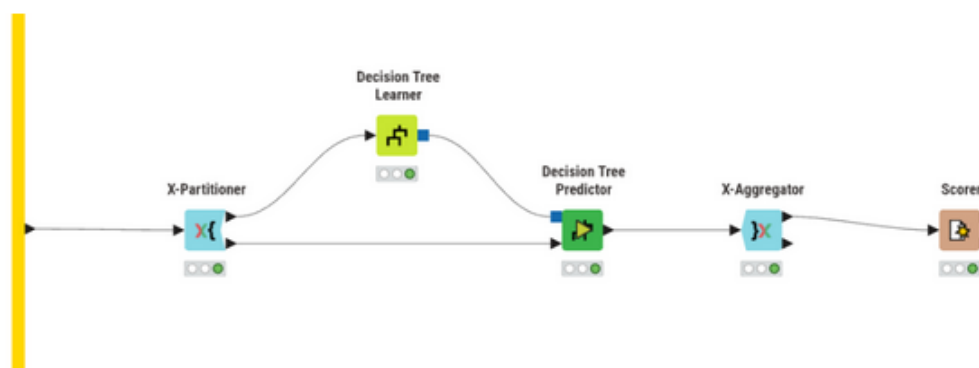
Figura 25: Metanode do modelo Decision Tree no KNIME
