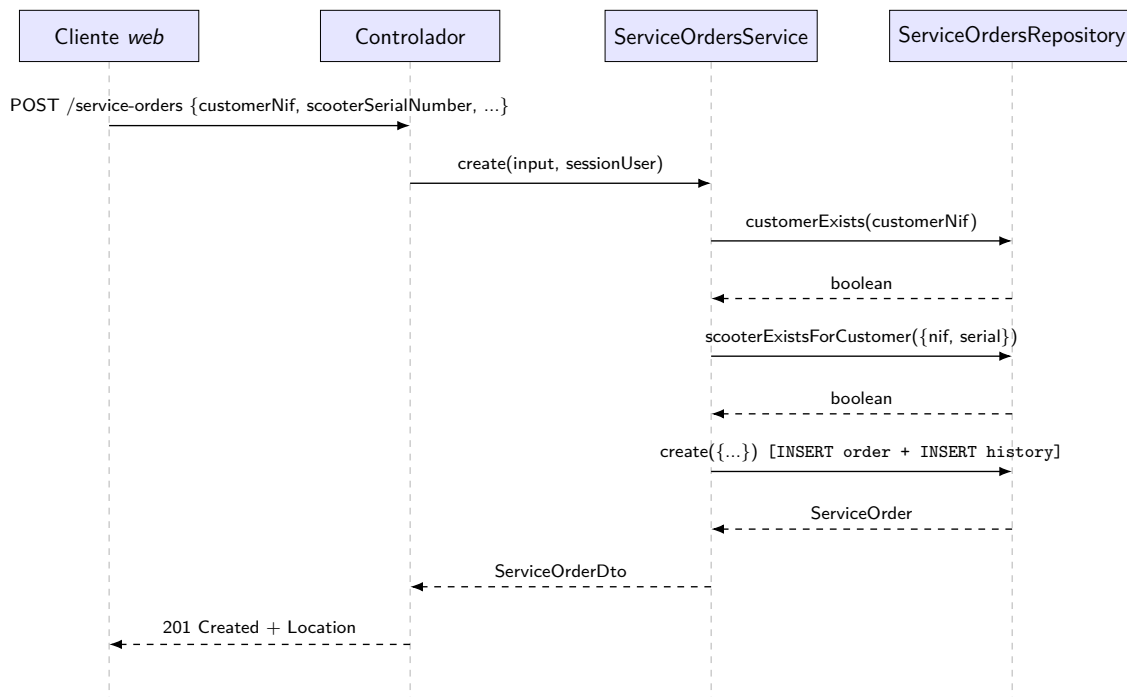
Figura 2.7: Diagrama de sequência da criação de ordem de serviço (POST /service-orders)
