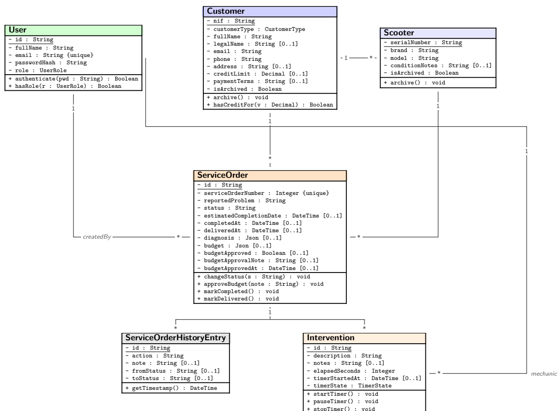
Figura 2.3: Diagrama de classes do subsistema operacional.
