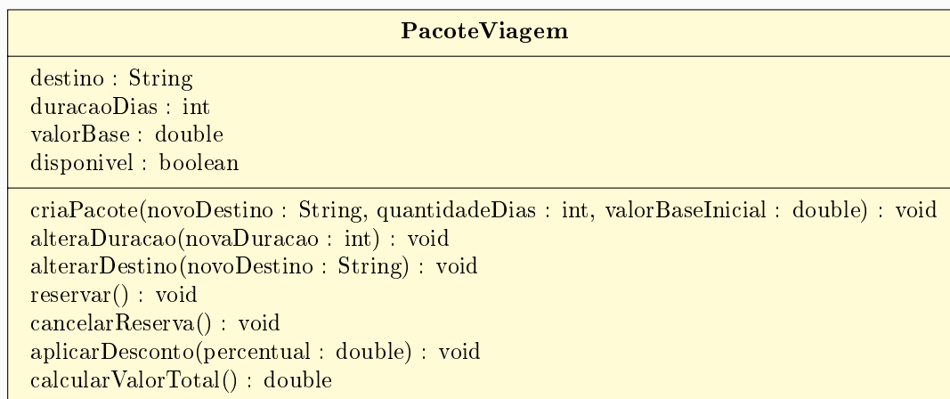
Figura 3: Diagrama UML da classe PacoteViagem.
