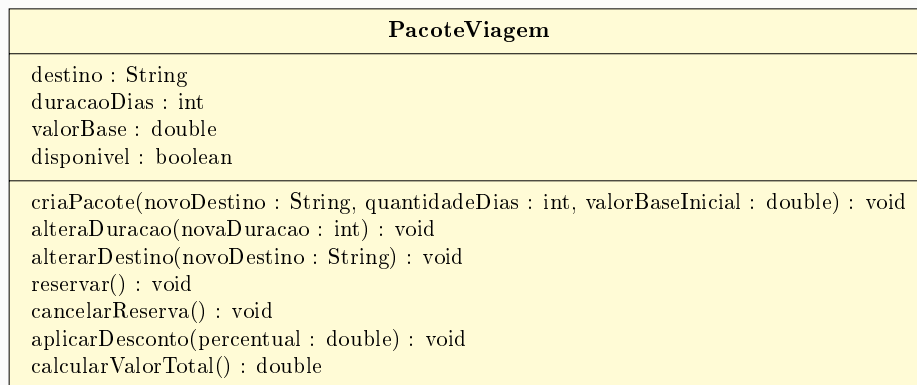
Figura 3: Diagrama UML da classe PacoteViagem.
