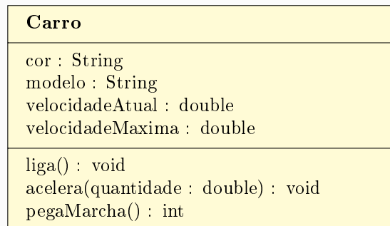
Figura 1: Diagrama UML da classe Carro.
