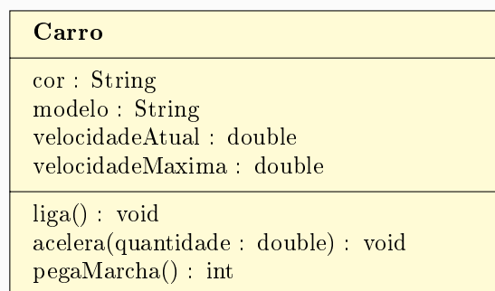
Figura 4.2: Diagrama UML da classe Carro.
