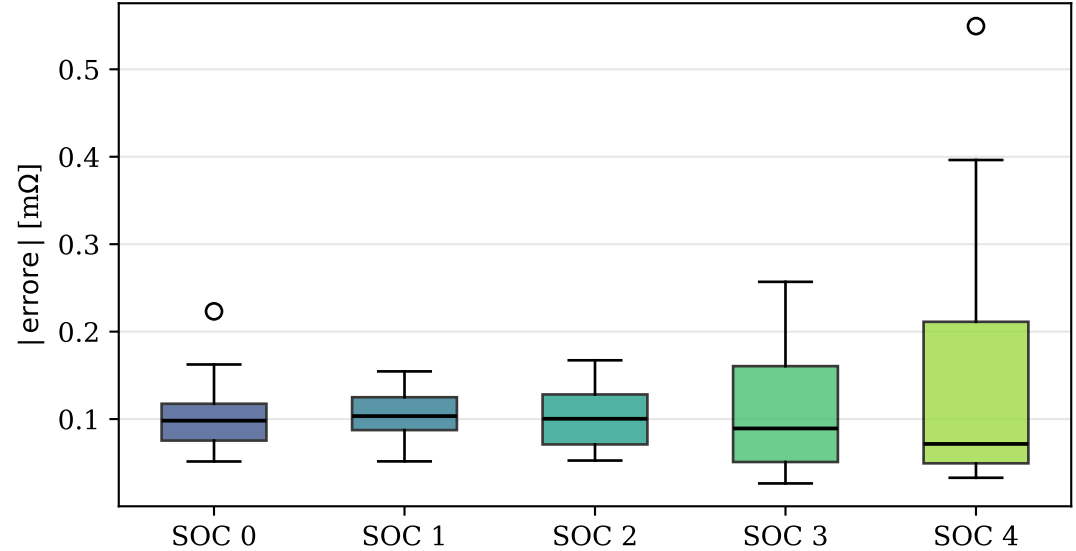
Task 1 — distribuzione dei residui per SOC (coppia esclusa: Aging=2, T = 22.5^{\circ}\text{C} , modello: K-Nearest Neighbors)
