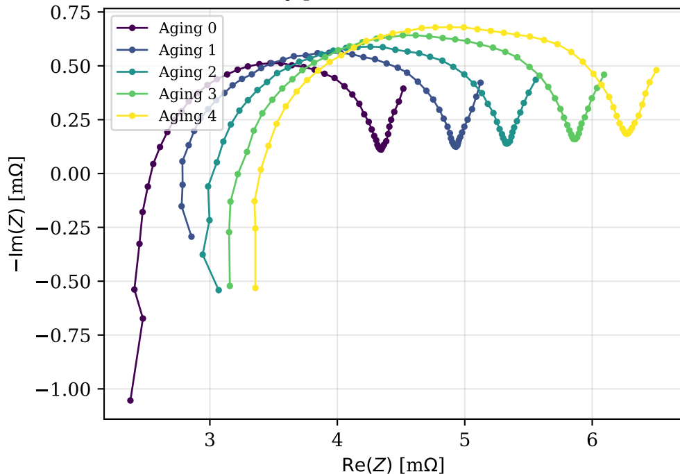
Evoluzione delle curve di Nyquist con l'invecchiamento ( T = 25\text{ }^{\circ}\text{C} , SOC = 2)
