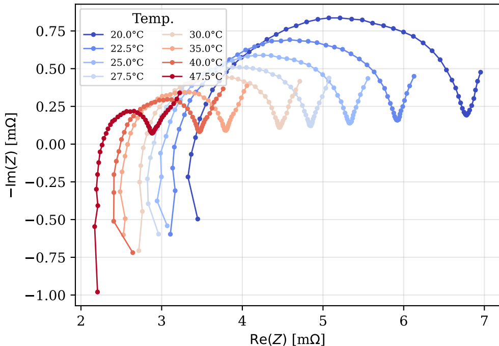
Curve di Nyquist a Aging = 2, SOC = 2
