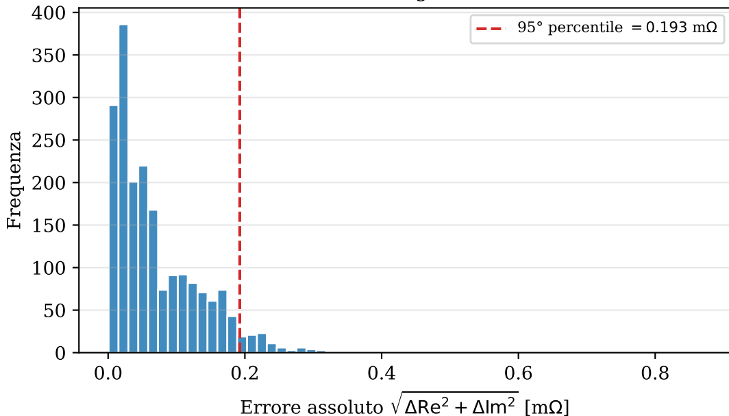
Task 3 — distribuzione degli errori sul fold di test
